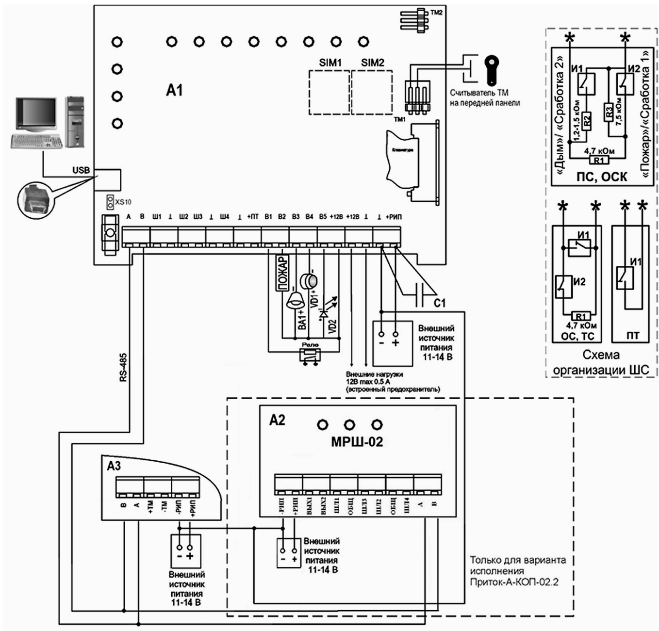
Рисунок 5 – Схема подключения
