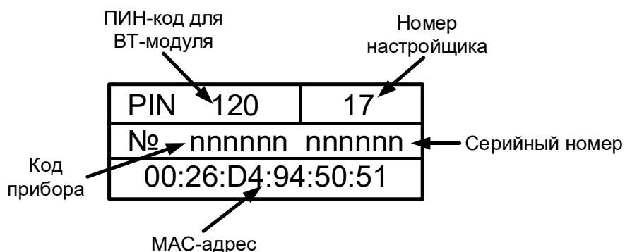
Рисунок 4.3 - Шильдик на плате Приток-А-КОП-04, Приток-А-КОП-05
