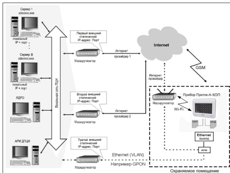
Рисунок 1.2 - Схема работы прибора с АРМ ПЦН
