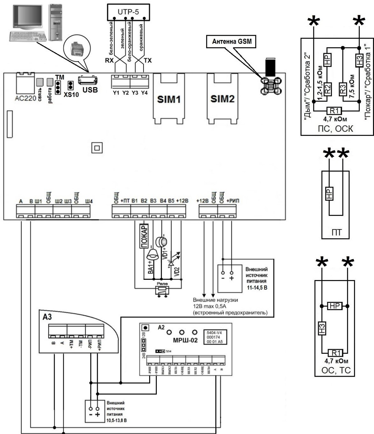
Рисунок А.4 – Схема подключения прибора Приток-А-КОП-02 (D)
