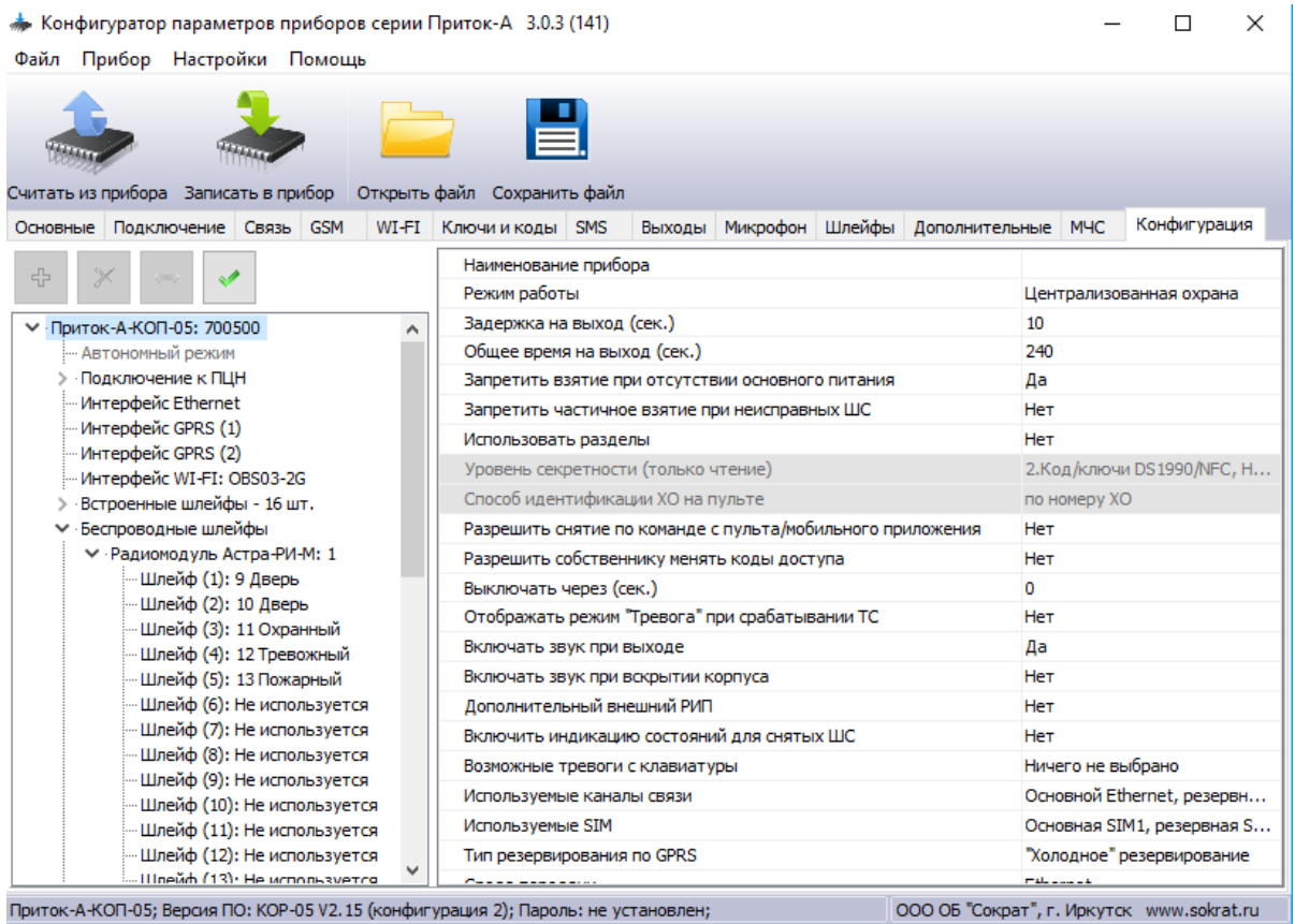
Рисунок Б.1 – Автоматически созданные беспроводные извещатели
