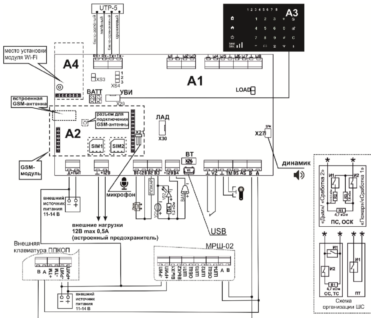
Рисунок А.7 – Схема подключения прибора версии Приток-А-КОП-04
