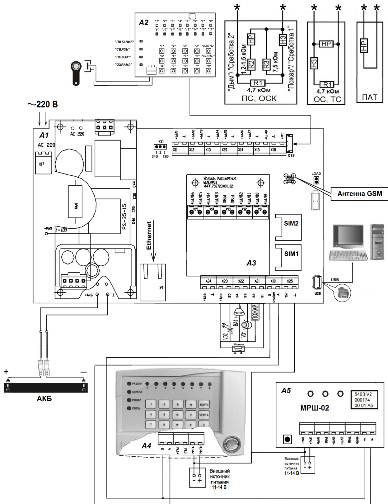
Рисунок А.1 – Схема подключения прибора версии Приток-А-КОП-01
