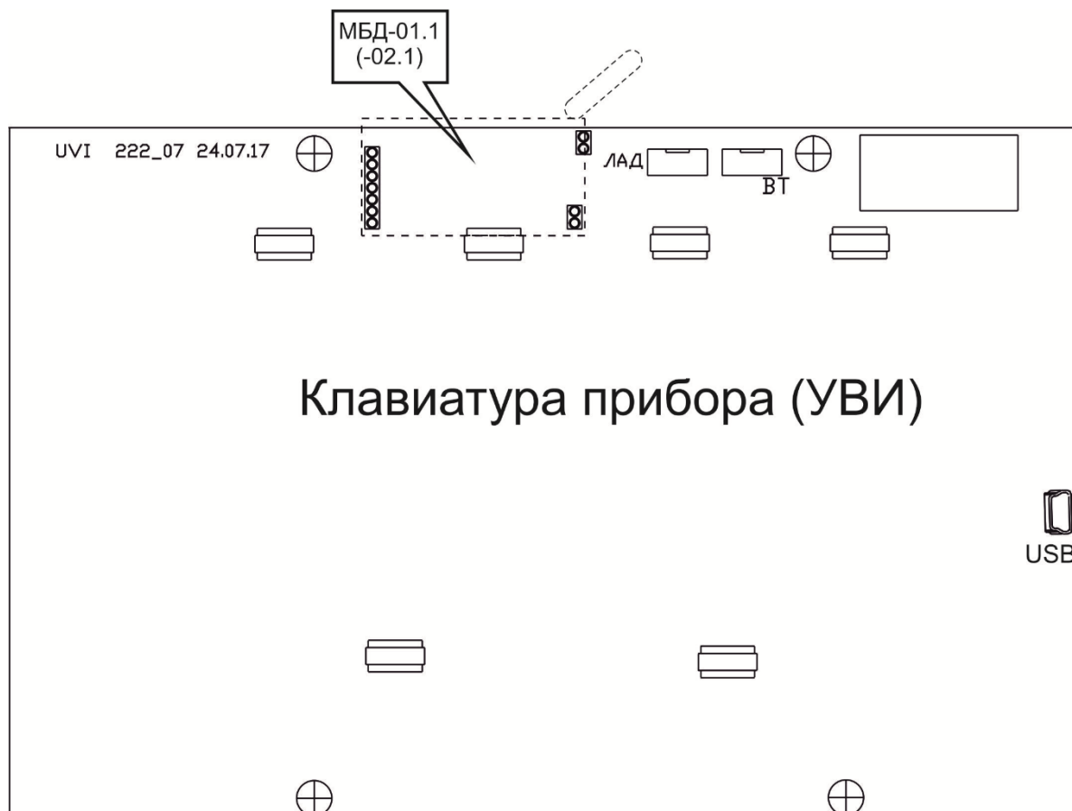
Рисунок Б.4 - Установка модулей беспроводных датчиков на плату УВИ
