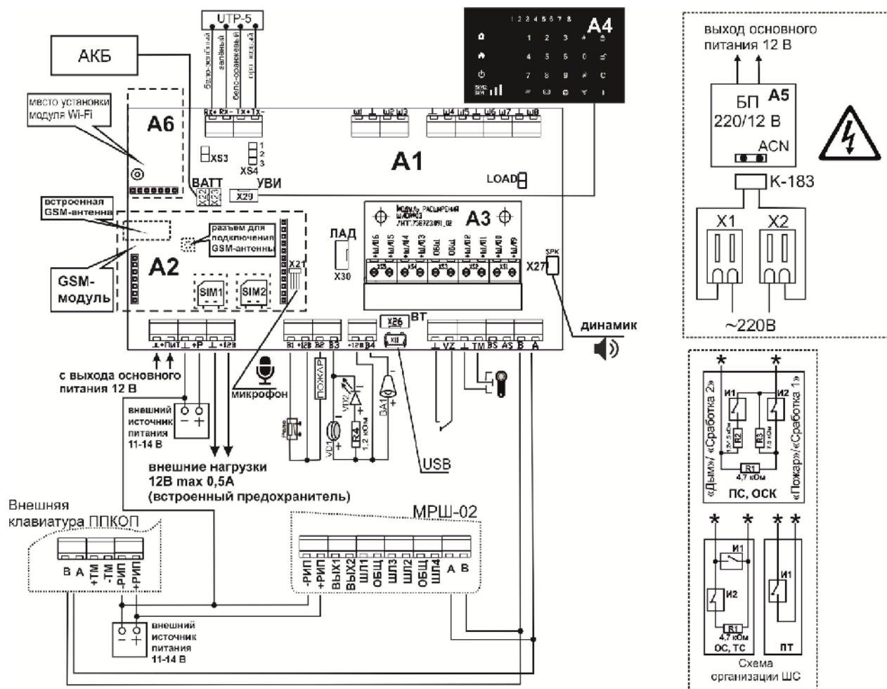
Рисунок А.9 – Схема подключения прибора версии Приток-А-КОП-05
