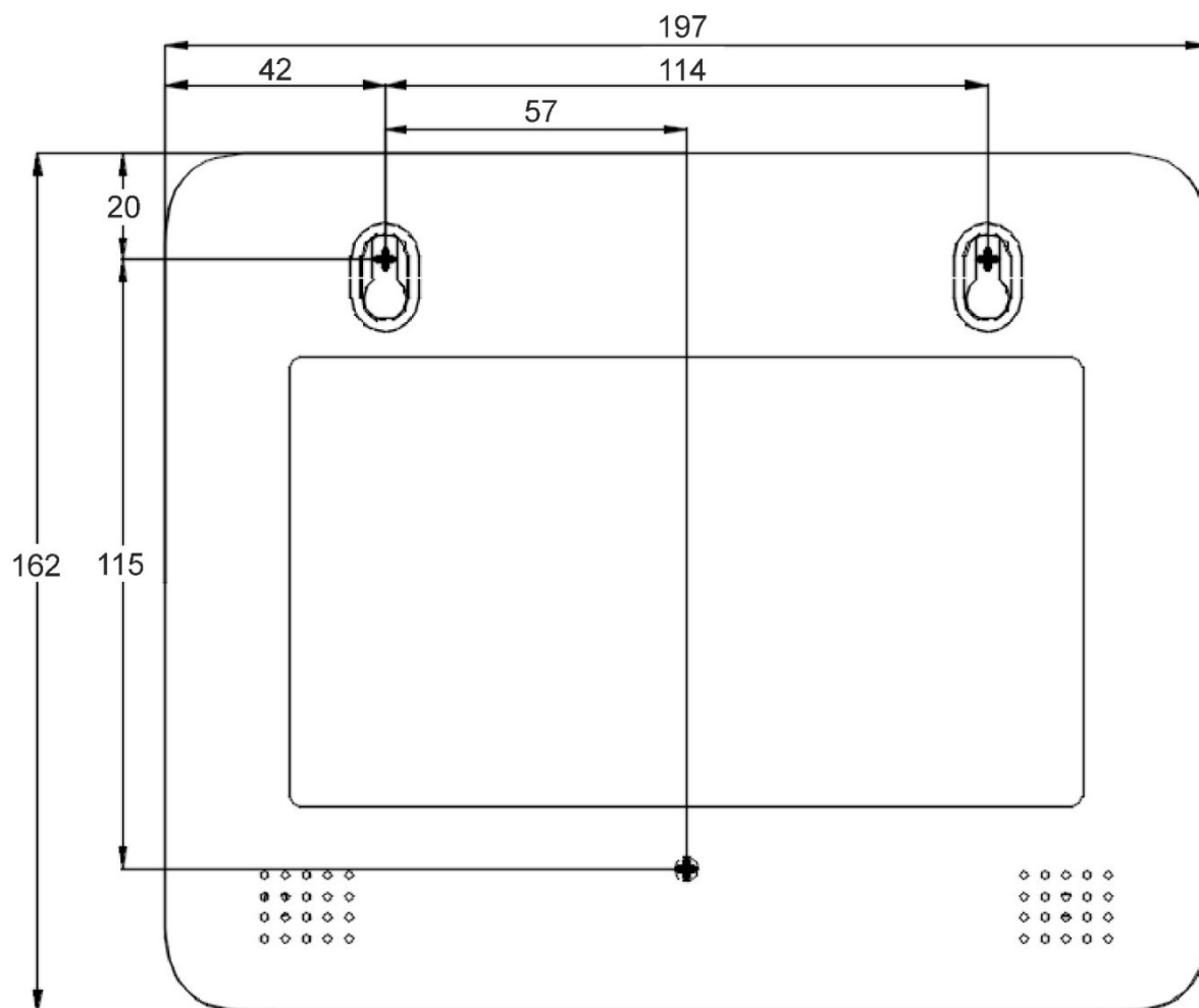
Рисунок Л.2 - Разметка отверстий для крепления прибора КОП-04 (вид со стороны передней панели).
