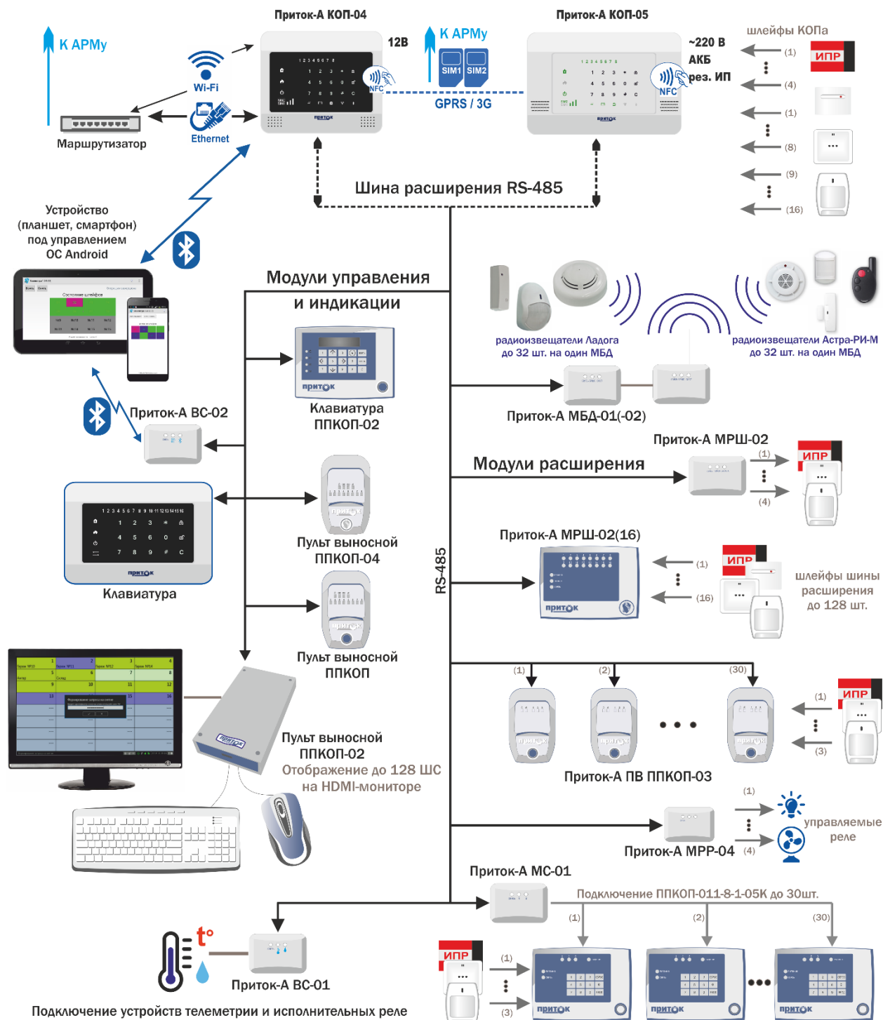
Рисунок В.1 - Подключаемые по шине расширения модули
