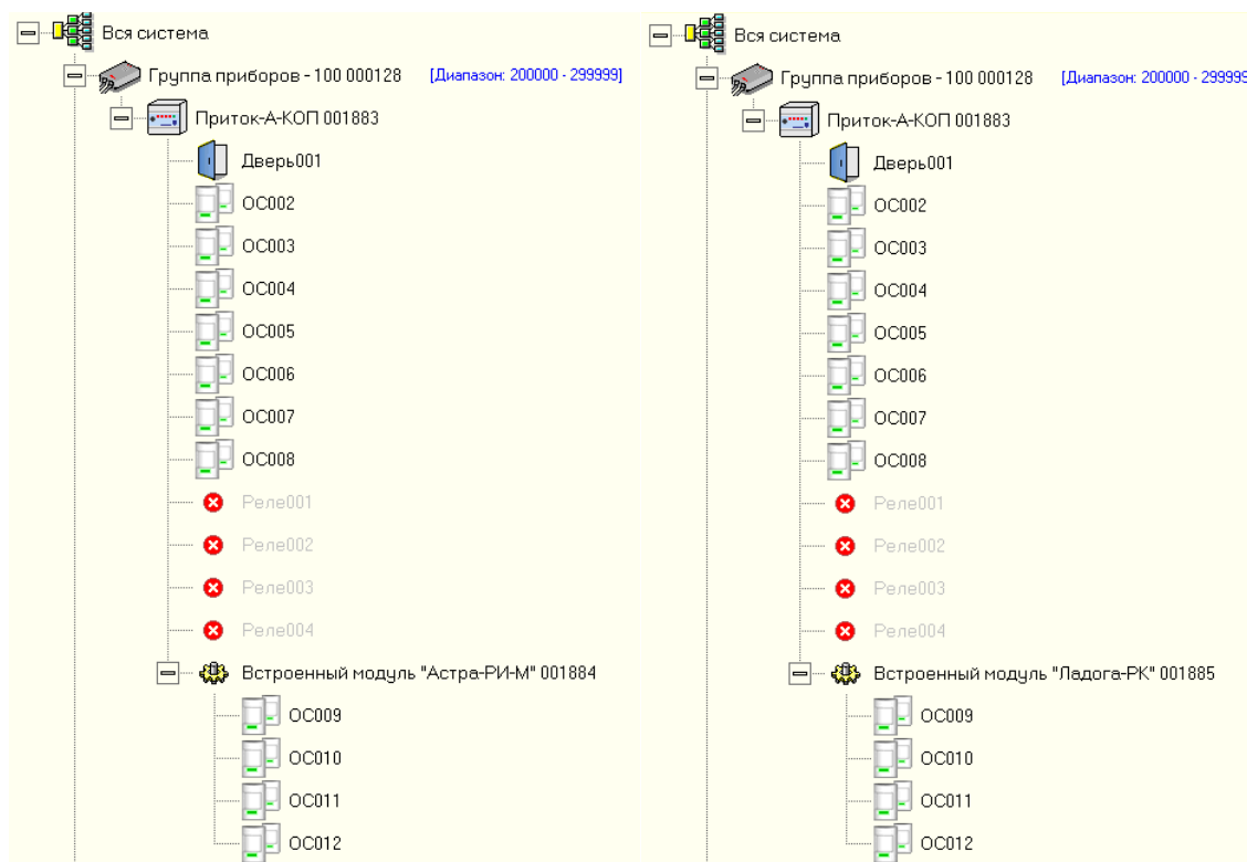
Рисунок Б.3 - Конфигурирование беспроводных шлейфов в АРМ Конфигуратор
