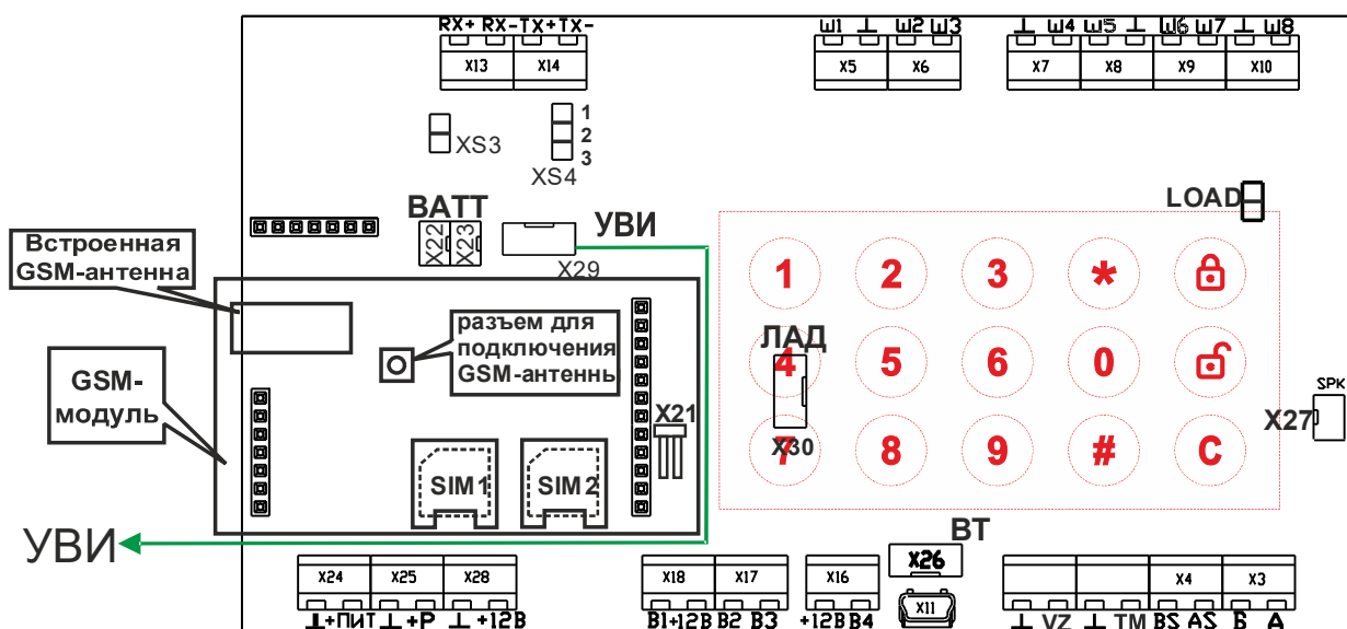
Рисунок 45 – Рекомендуемая укладка кабеля между платой УВИ и платой прибора
