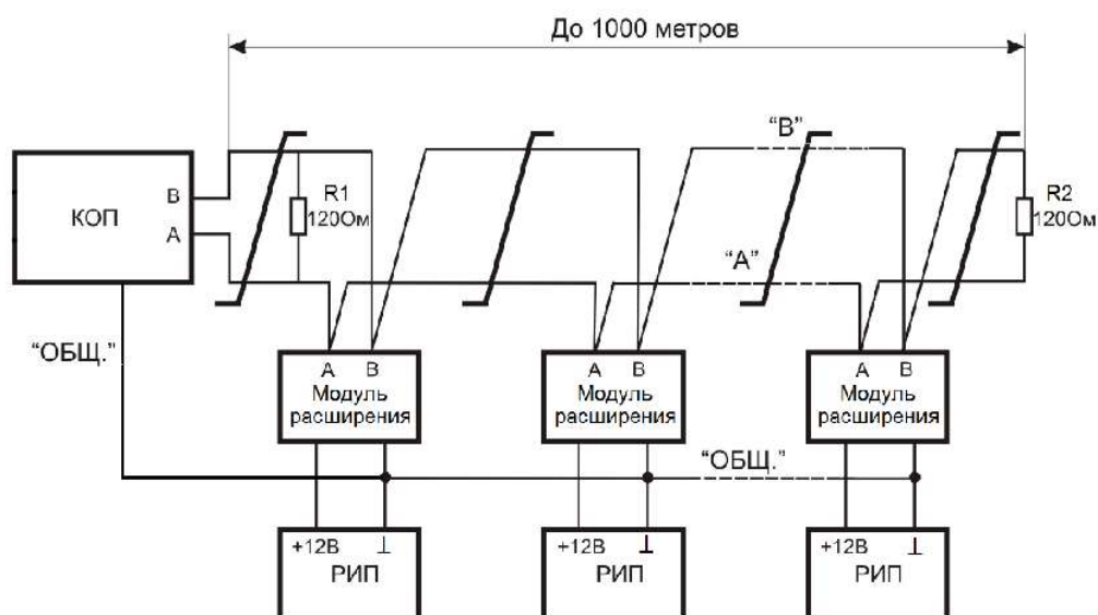
Рисунок 49 – Схема подключения приборов к линиям интерфейса RS-485
