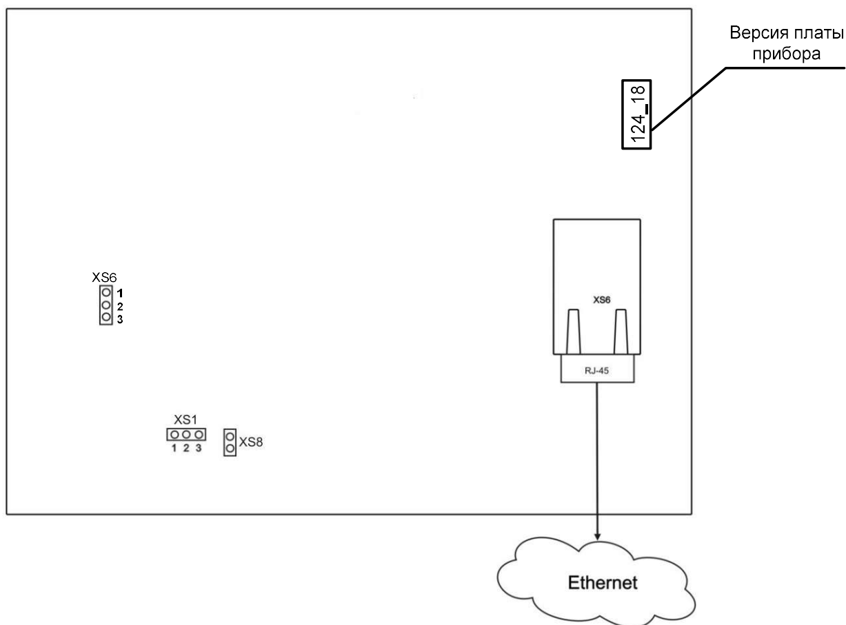
Рисунок 39 – Схема подключения прибора Приток-А-КОП-02
