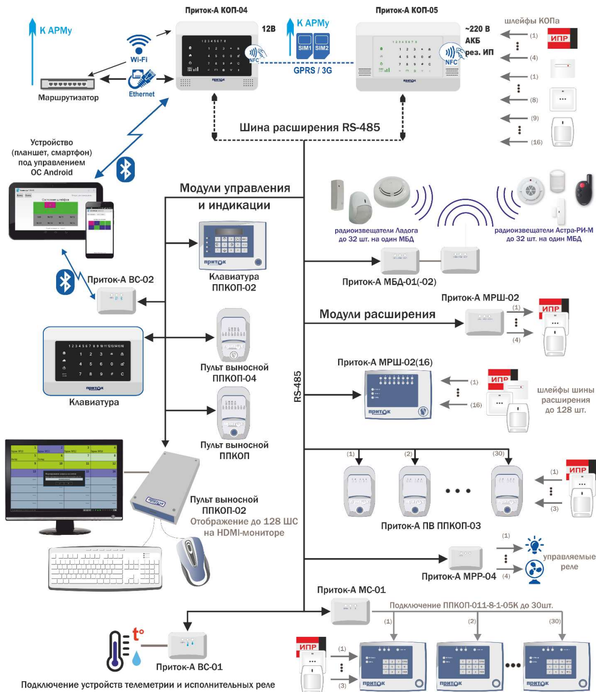
Рисунок 54 – Подключаемые по шине расширения модули
