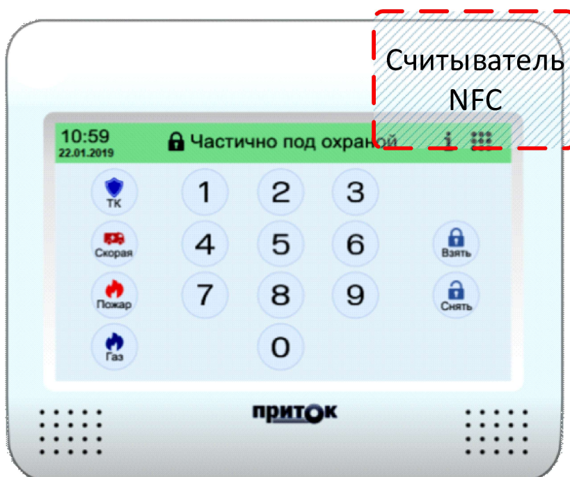
Рисунок 60 – Внешний вид прибора
