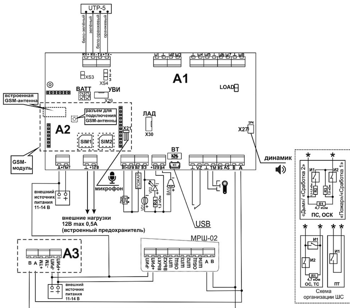
Рисунок 47 – Схема подключения прибора Приток-А-КОП-04 (D)
