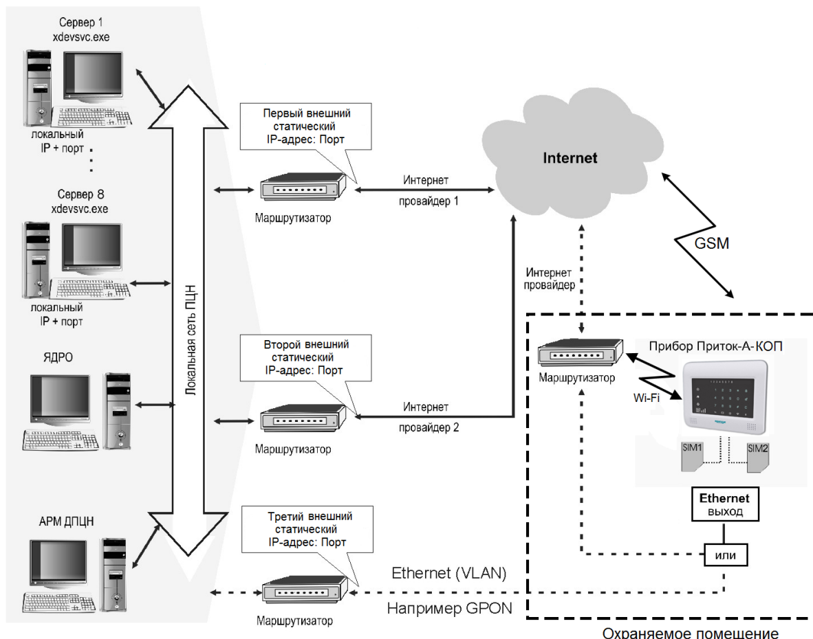
Рисунок 2 – Схема работы прибора с АРМ ПЦН
