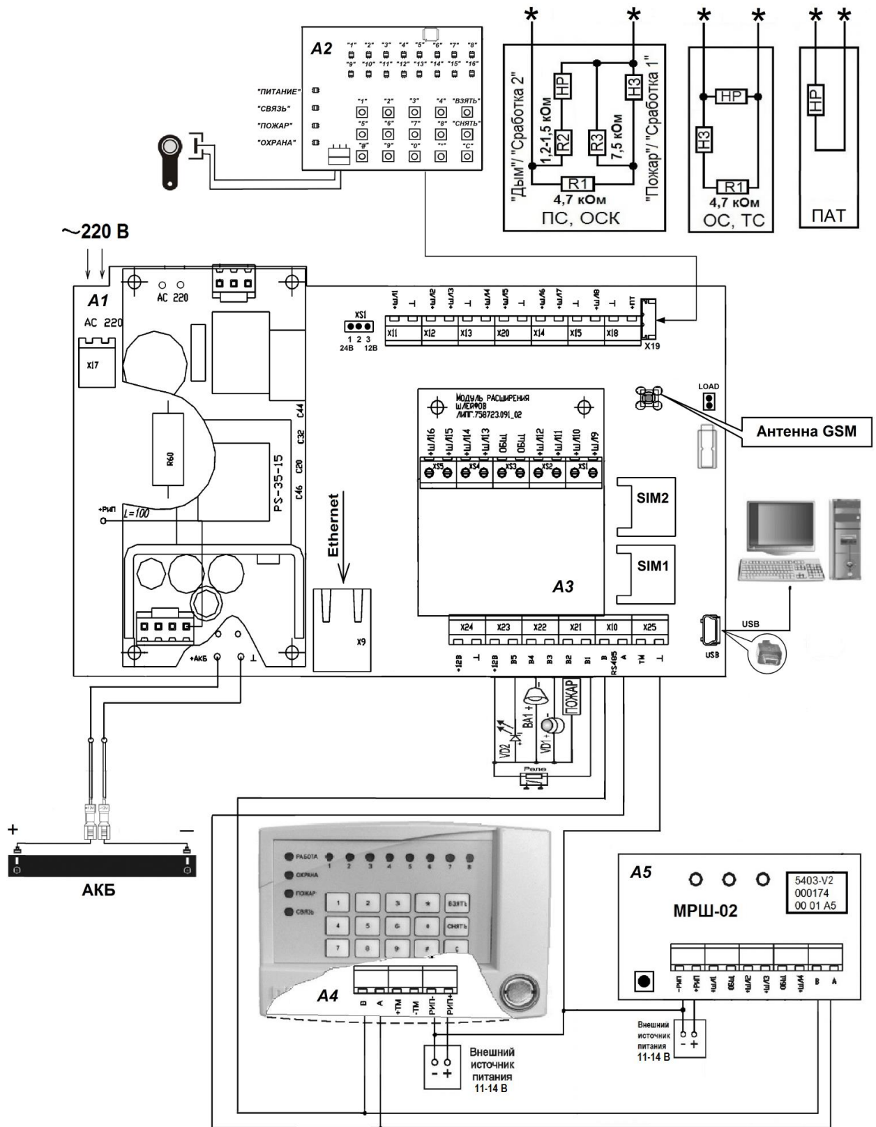
Рисунок 36 – Схема подключения прибора версии Приток-А-КОП-01
