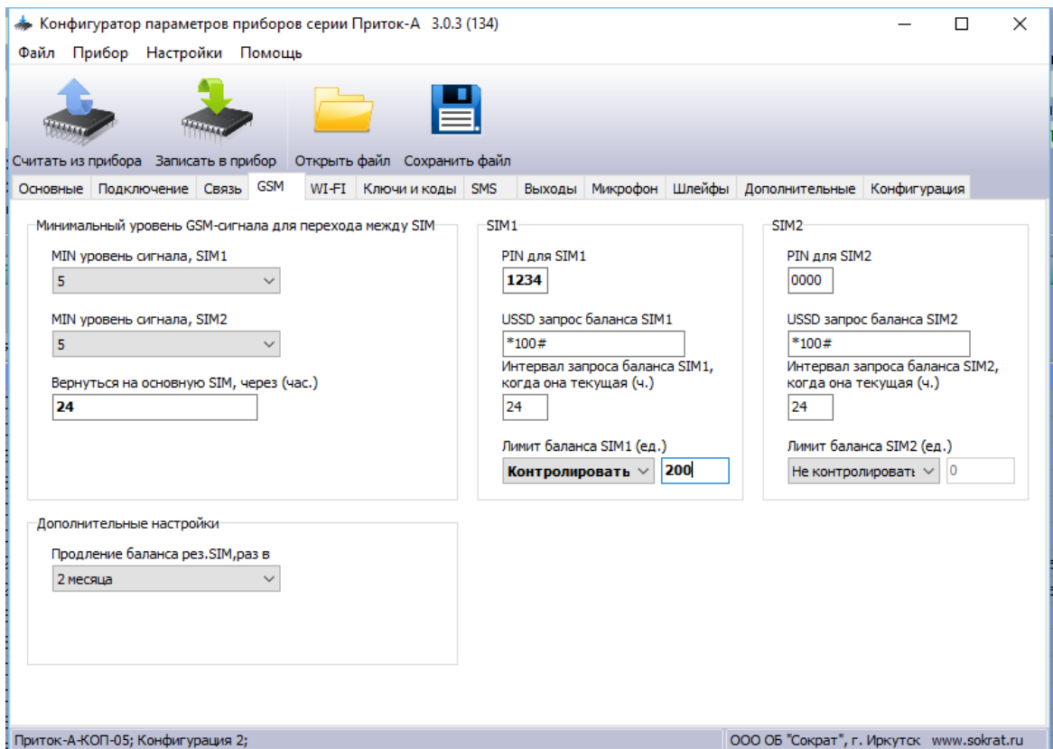
Рисунок 10 – Вкладка «Параметры GSM»
