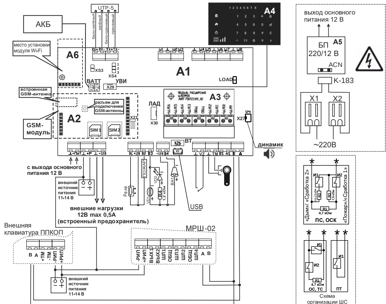
Рисунок 44 – Схема подключения прибора версии Приток-А-КОП-05
