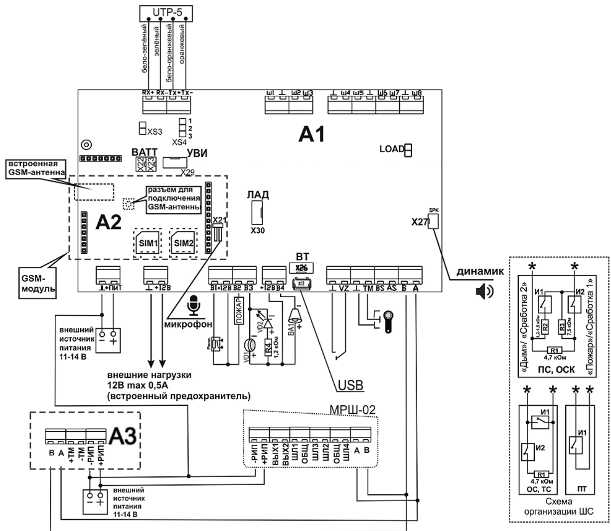
Рисунок 47 – Схема подключения прибора версии Приток-А-КОП-04 (D)
