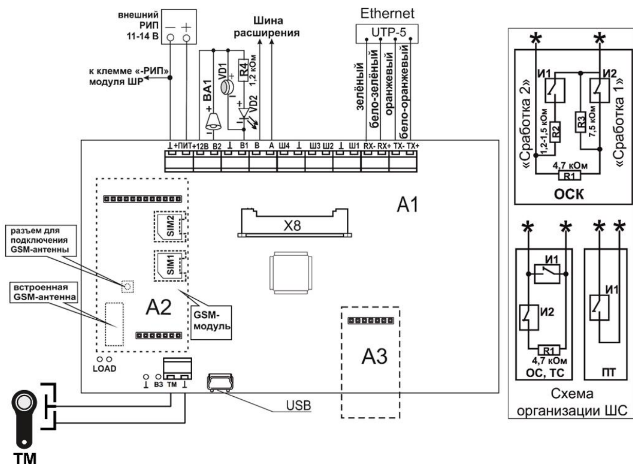
Рисунок 40 – Схема подключения Устройства оконечного объектового Приток-А-КОП-02.4
