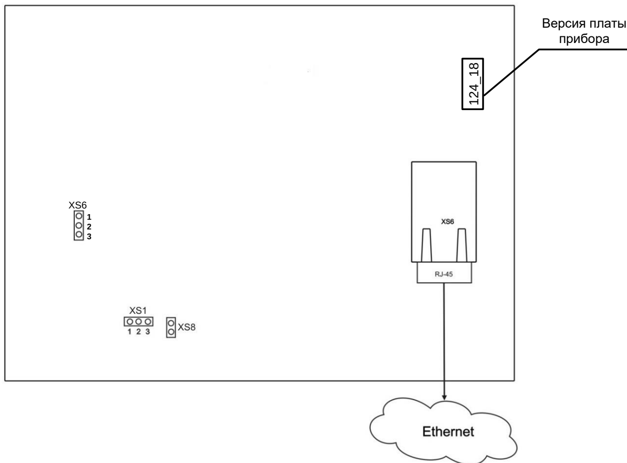
Рисунок 38 – Схема подключения прибора версии Приток-А-КОП-02. Тыльная сторона
