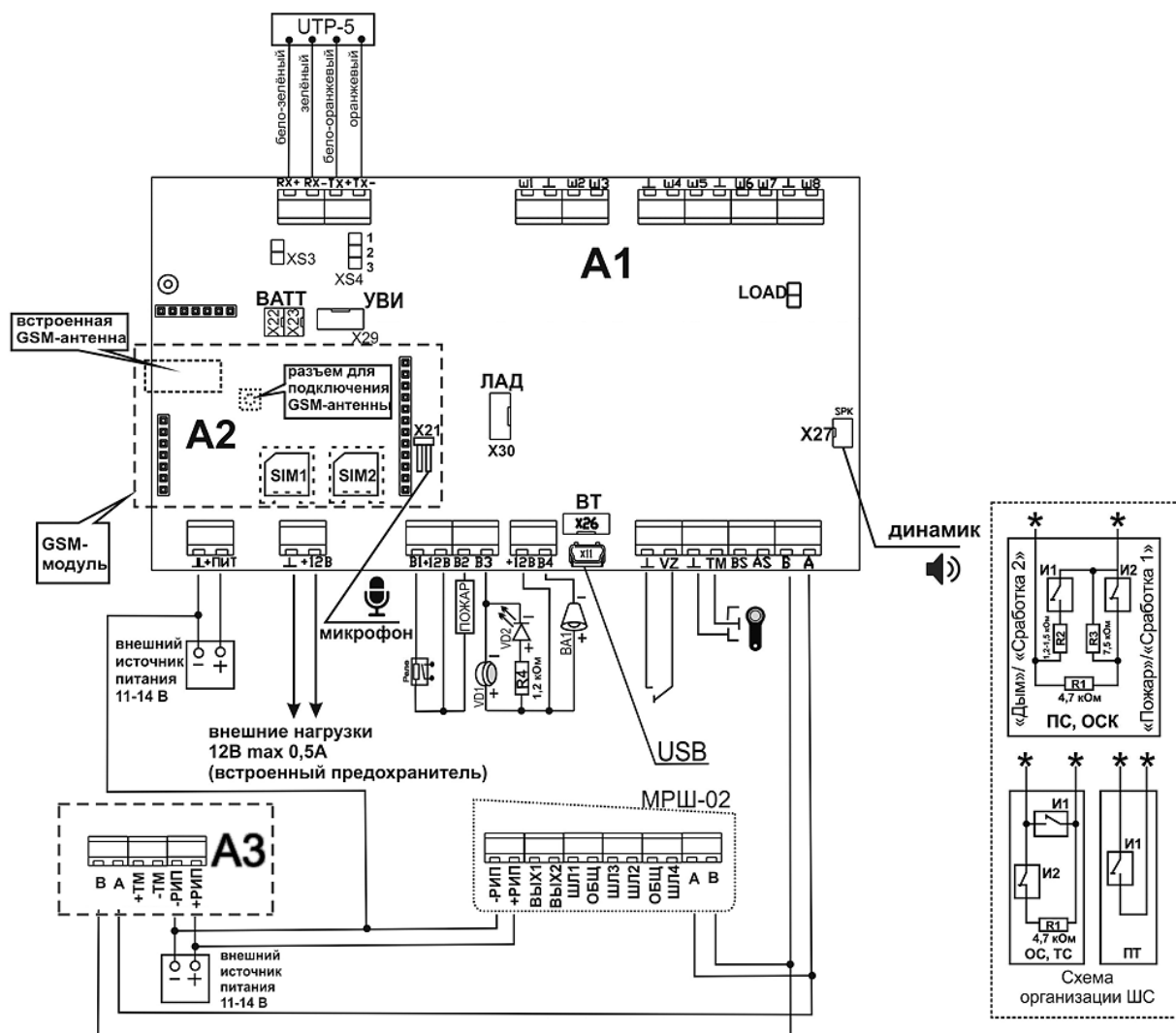
Рисунок 47 – Схема подключения прибора версии Приток-А-КОП-04 (D)
