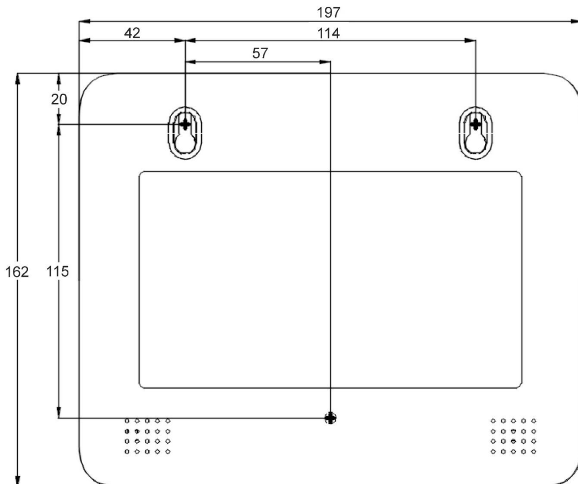
Рисунок 54 – Разметка отверстий для крепления прибора КОП-04 (вид со стороны передней панели).
