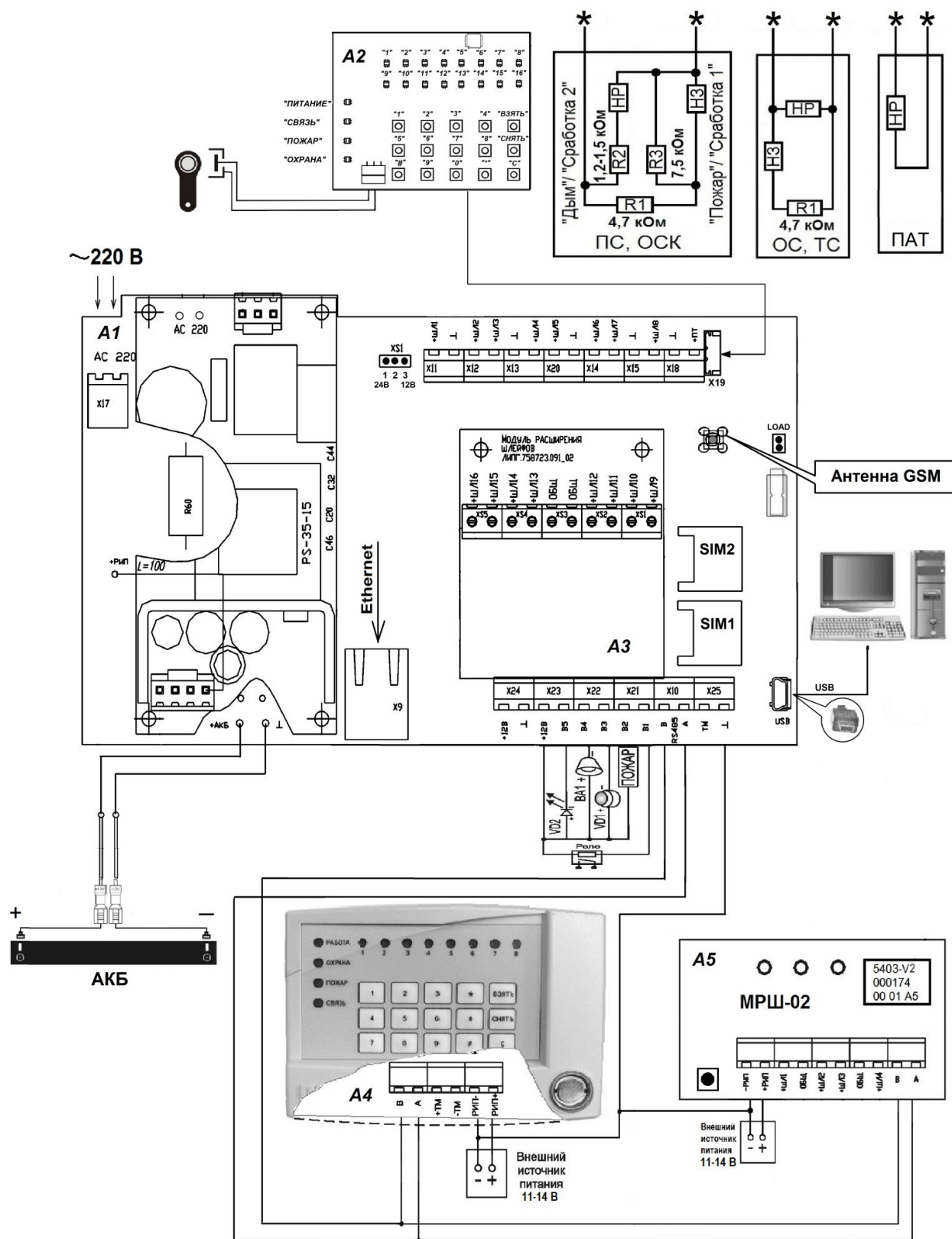
Рисунок 36 – Схема подключения прибора версии Приток-А-КОП-01
