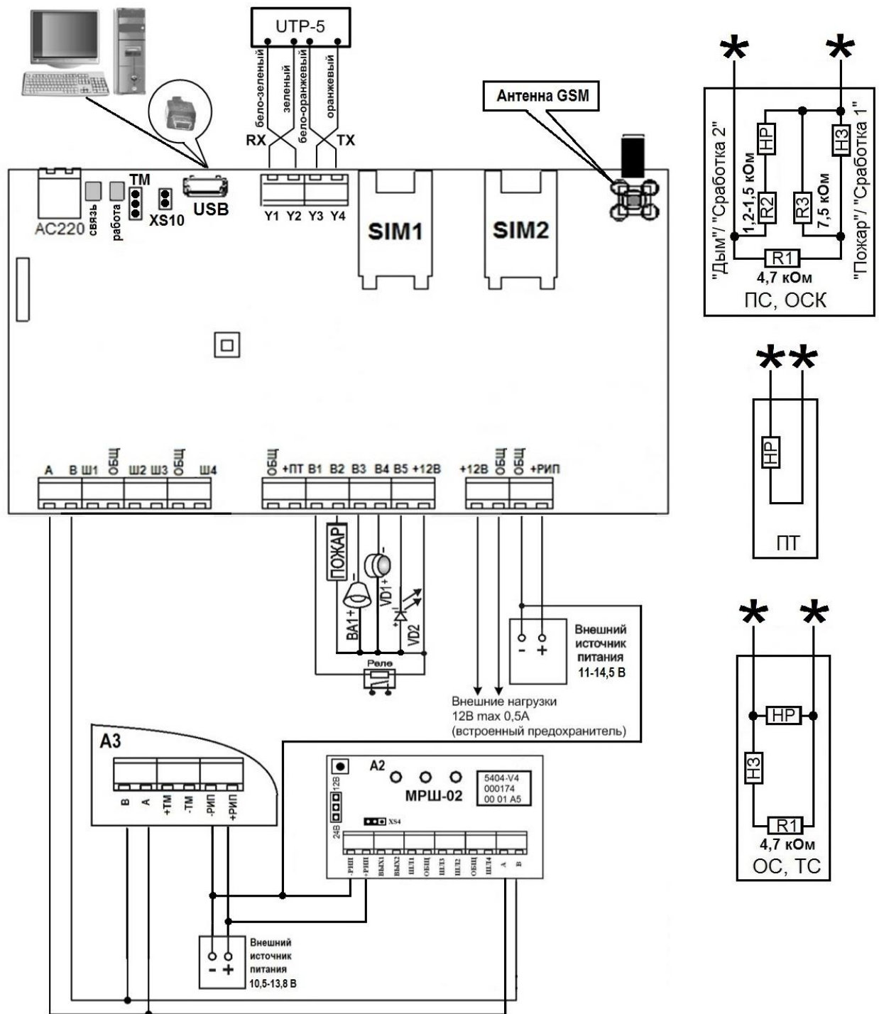
Рисунок 39 – Схема подключения прибора Приток-А-КОП-02 (D)
