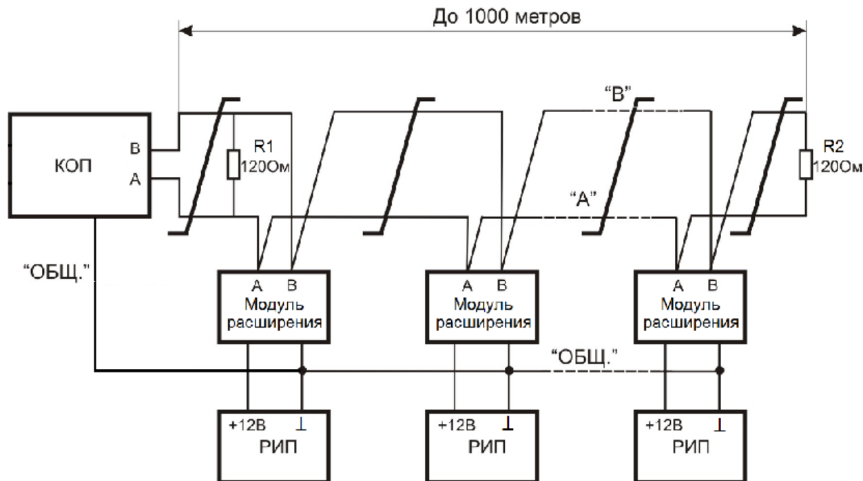
Рисунок 46 – Схема подключения приборов к линиям интерфейса RS-485
