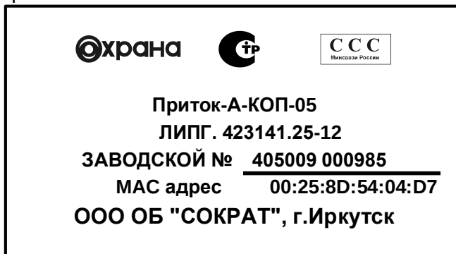
Рисунок 32 – Шильдик на корпусе
