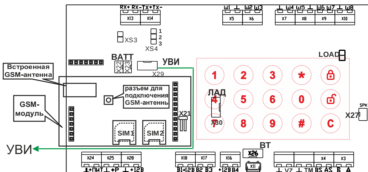
Рисунок 43 – Рекомендуемая укладка кабеля между УВИ и платой прибора
