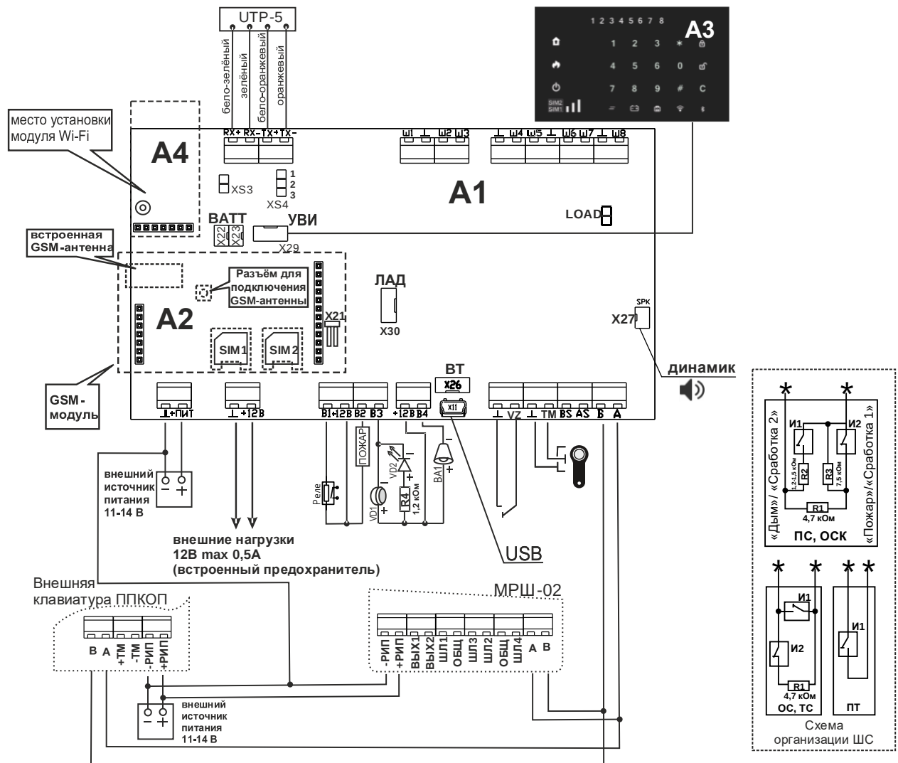
Рисунок 42 – Схема подключения прибора версии Приток-А-КОП-04
