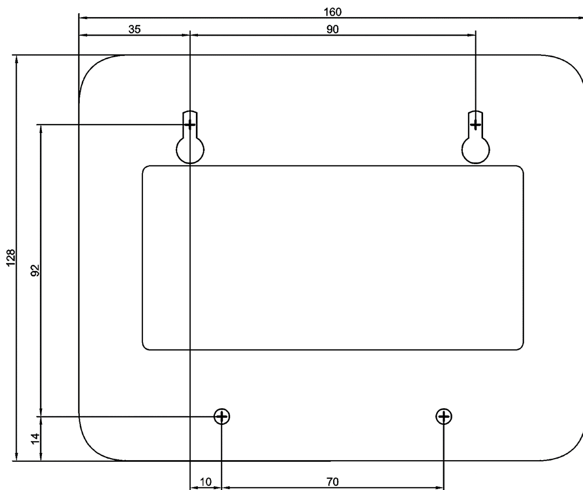
Рисунок 56 – Разметка отверстий для крепления прибора КОП-02.4 (вид со стороны передней панели)
