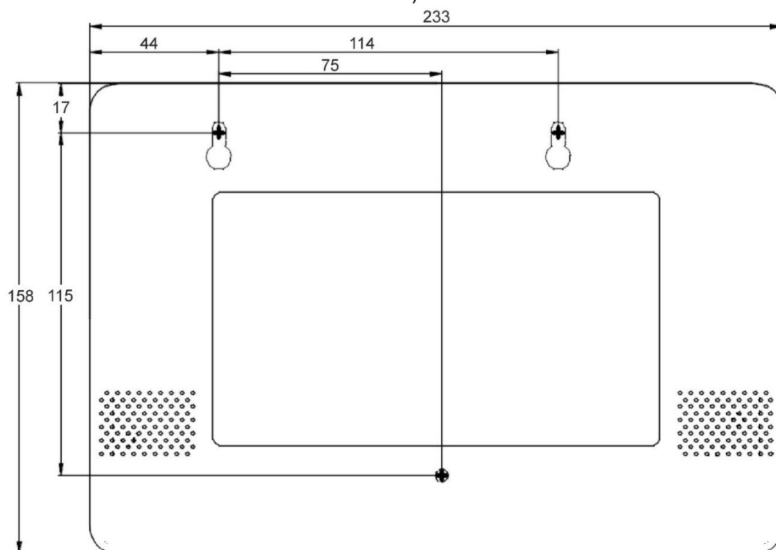
Рисунок 55 – Разметка отверстий для крепления прибора КОП-05 (вид со стороны передней панели)
