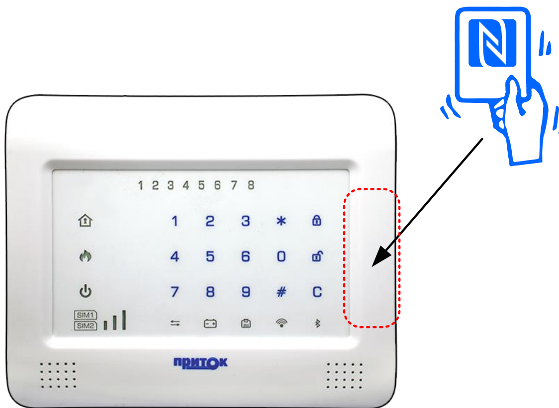
Рисунок 45 – Расположение бесконтактного считывателя
