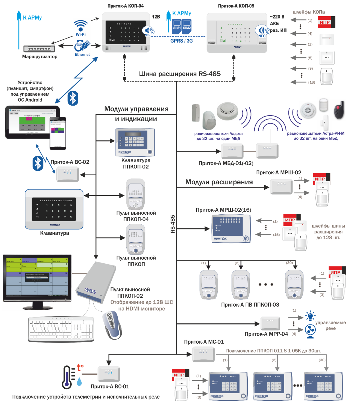
Рисунок 52 – Подключаемые по шине расширения модули
