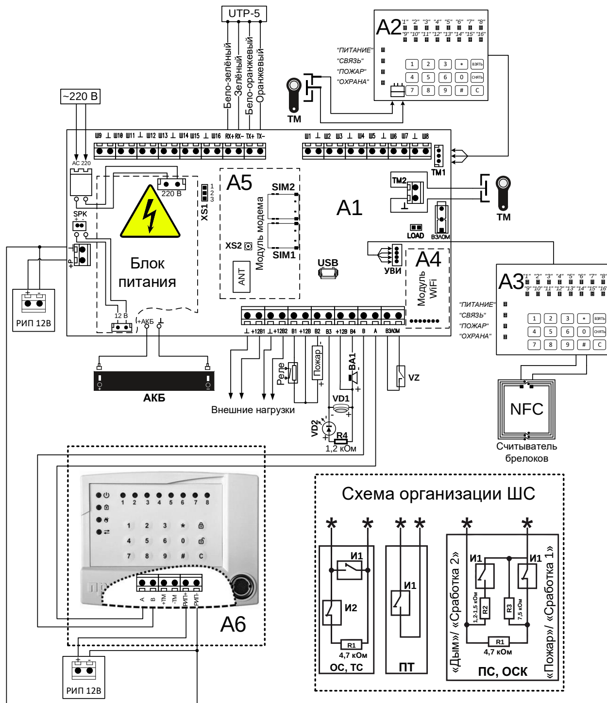
Рисунок 41 – Схема подключения прибора Приток-А-КОП-03 и Приток-А-КОП-03 NFC
