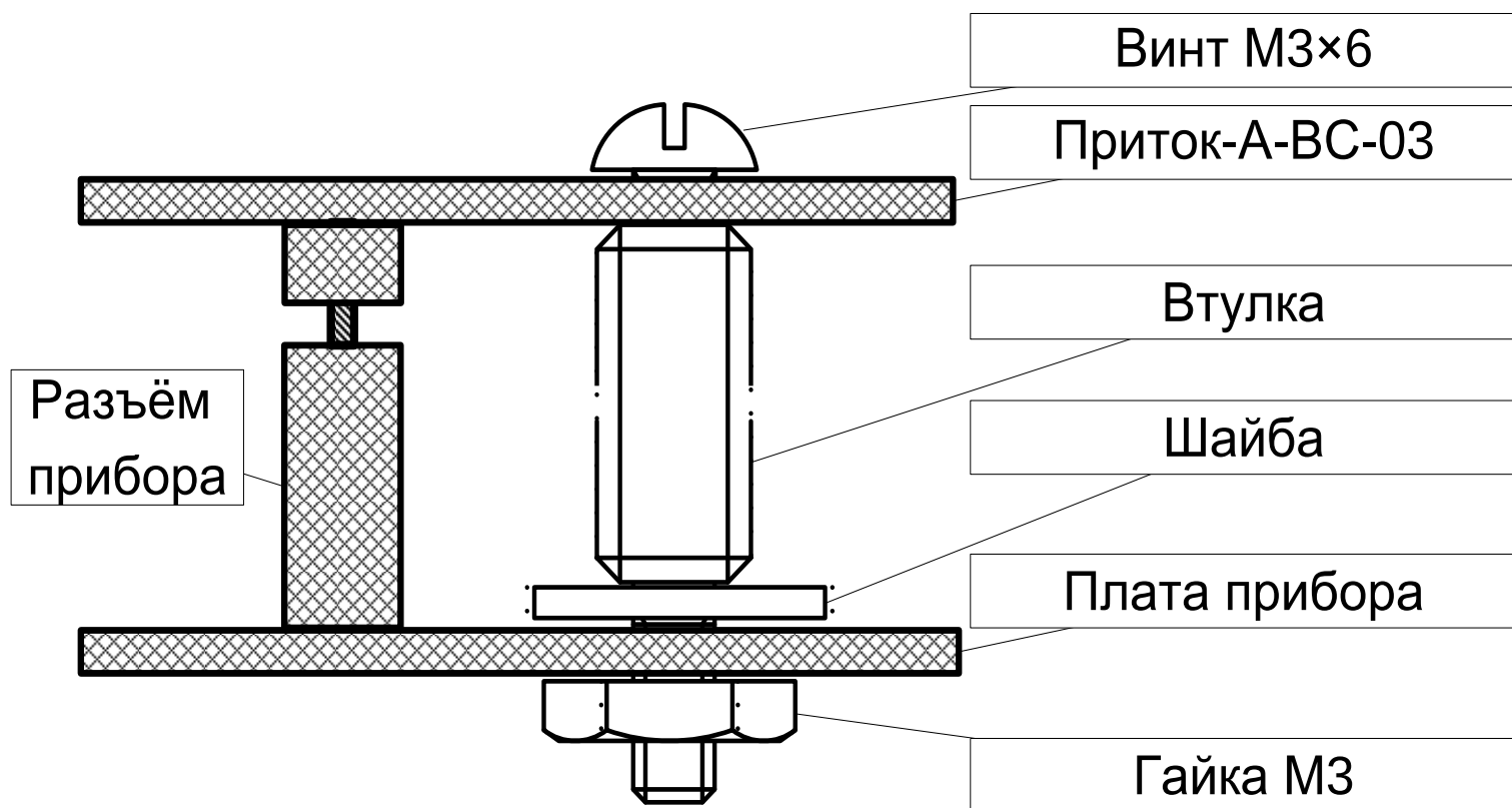
Рис. 1. Схема монтажа модуля
