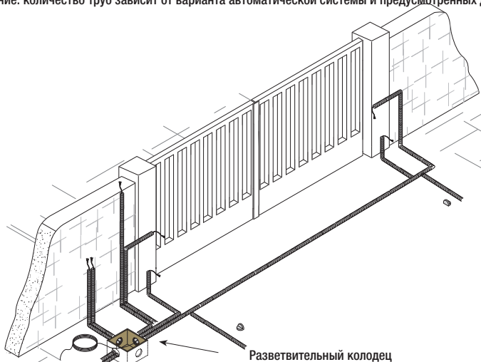
Разветвительный колодец
