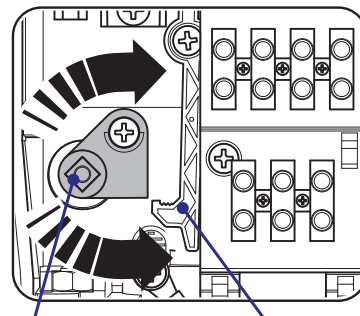
Рычаг разблокировки
