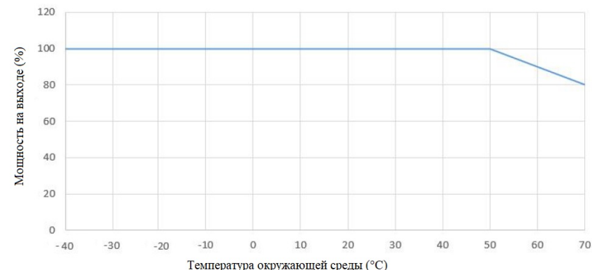
Зависимость выходной мощности от температуры окружающей среды
