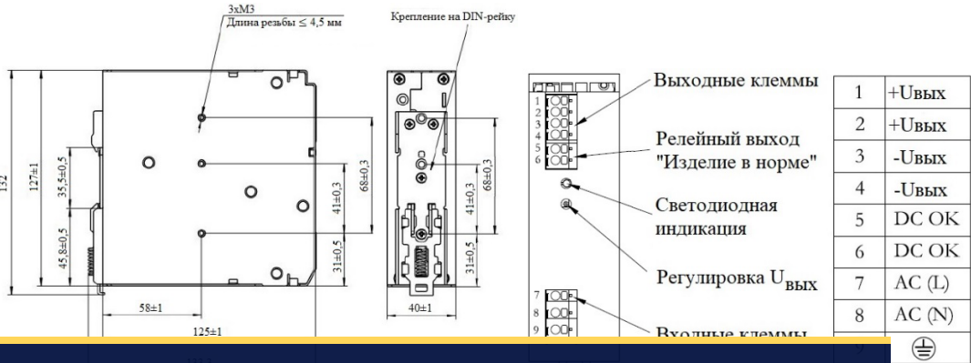
Габаритные размеры изделия
