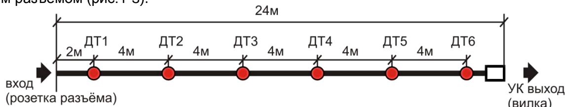
Рис.1. Расположение тепловых датчиков (ДТ) в кабельном хвосте ProCab® ИП101-1-Р-МТ.
