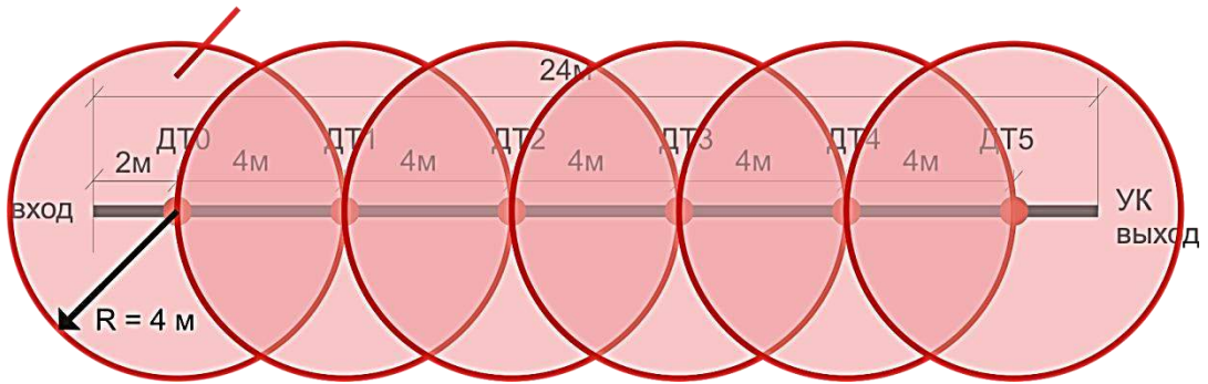
Рис.7. Зона мониторинга тепловыми датчиками КХ ProCab® ИП101-1-Р-МТ.
