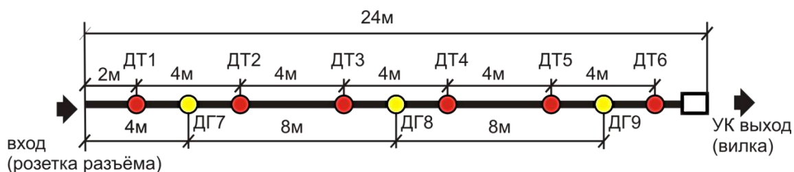
Рис.3. Расположение тепловых датчиков (ДТ) и газовых датчиков (ДГ) в кабельном хвосте ProCab® ИП101/435-2-Р-МТ (газ СО, тепло).
