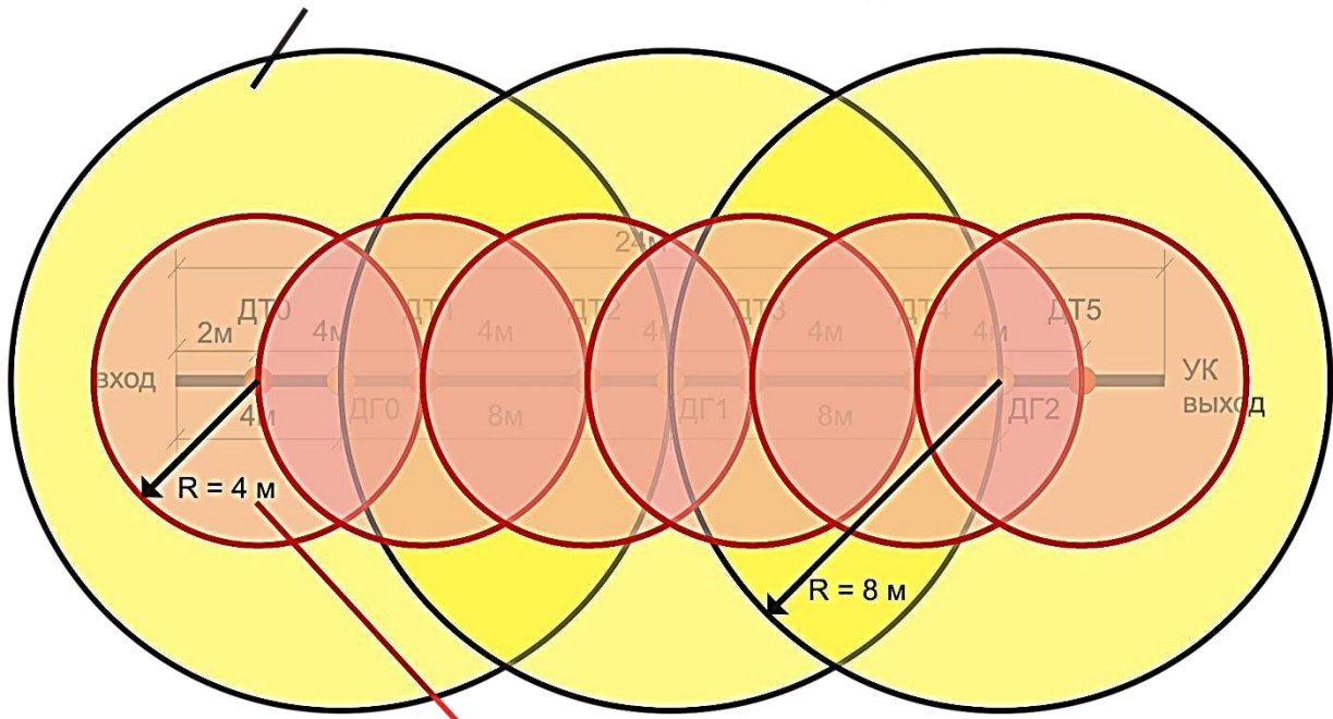
Рис.9. Зона мониторинга газовыми и тепловыми датчиками КХ ProCab® ИП101/435-2-Р-МТ.
