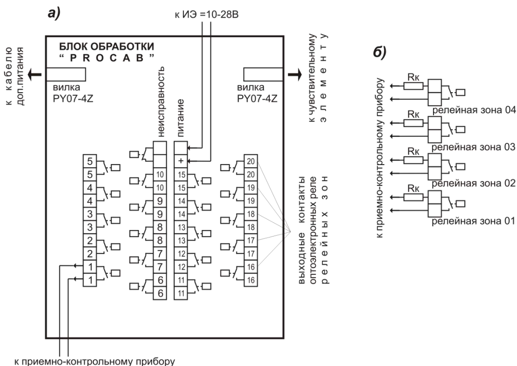
Рис.19. Внешние соединения блока обработки извещателя.
