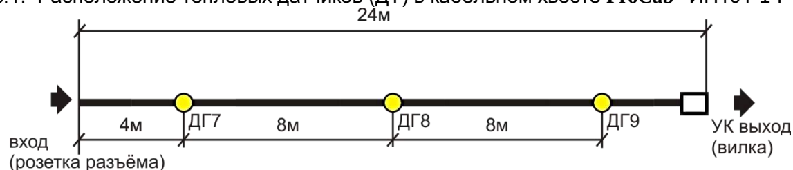
Рис.1. Расположение тепловых датчиков (ДТ) в кабельном хвосте ProCab® ИП101-1-Р-МТ.
