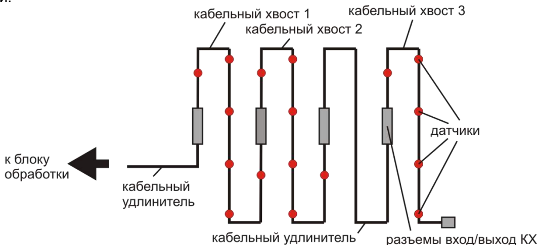
Рис.10. Чувствительный элемент извещателя из трёх КХ и двух кабельных удлинителей.
