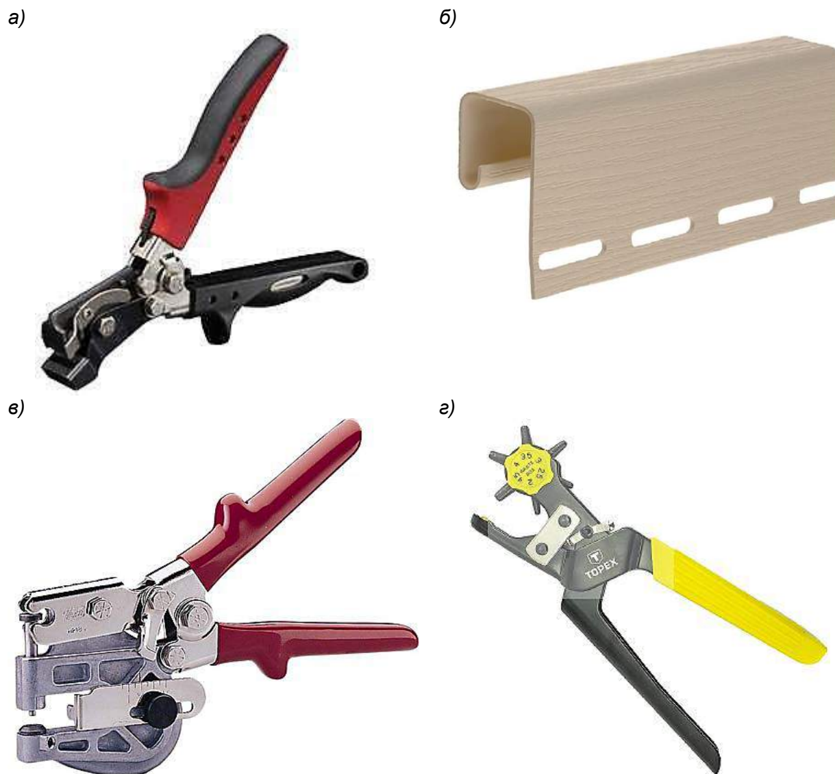
Рис.16. Инструменты для просечки отверстий в крышке кабель-канала.
