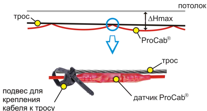
Рис.13. Монтаж ЧЭ ProCab® на тросу.
