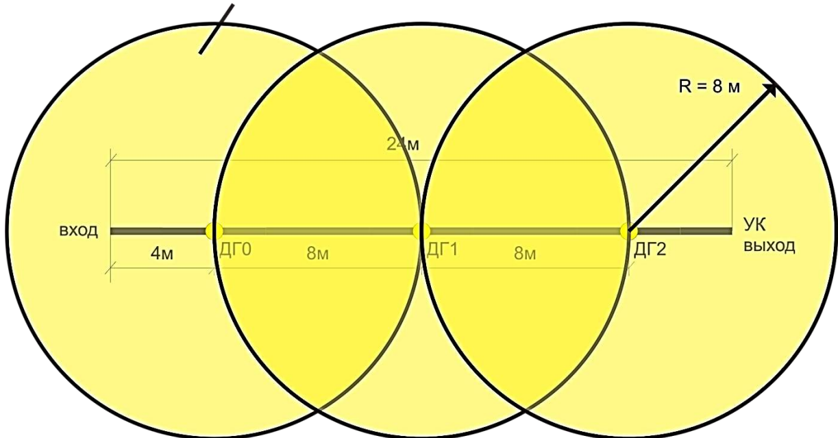
Рис.8. Зона мониторинга газовыми датчиками КХ ProCab® ИП435-6-МТ.
