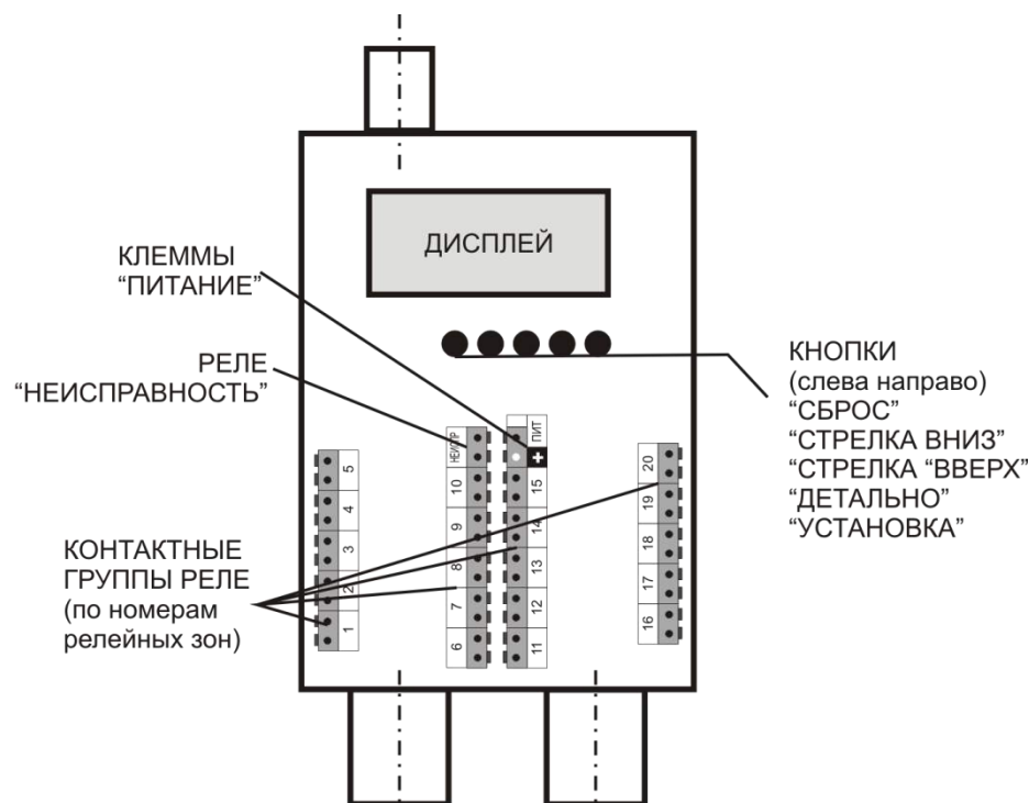
Рис.20. Расположение кнопок и клеммников блока обработки (крышка БО снята)
