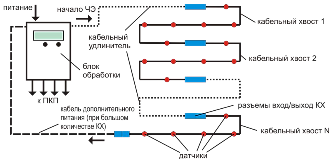
Рис. 12. Соединения составных частей извещателя ProCab®.
