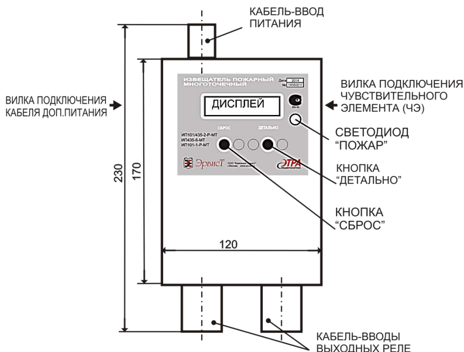
Рис. 18. Габариты БО и расположение подключений к блоку обработки.
