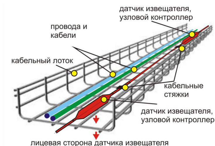
Рис.15. Прокладка ЧЭ ProCab® в решётчатых кабельных лотках.
