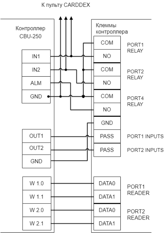
Электронные проходные CARDDEX, контроллер турникета CBU-250 (CBU-150/250).
