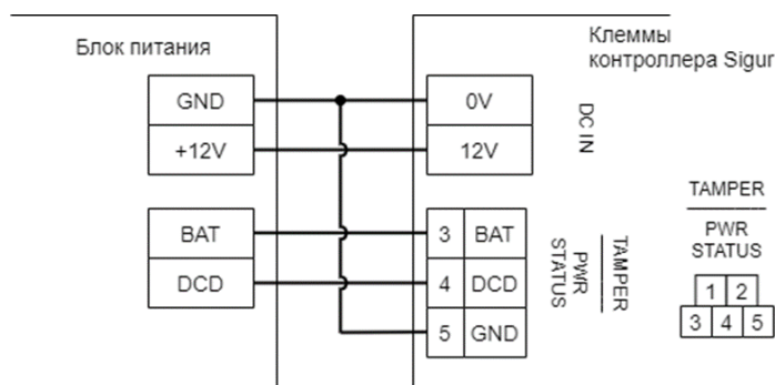
Подключение питания к контроллеру.
