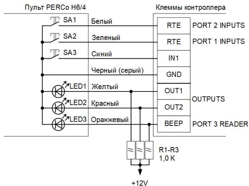
Пульт управления PERCo-КТ02 и КТ05.3.
