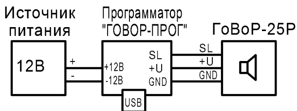
Рис. Б.5 Схема подключения GoBoP-25P к программатору GoBoP-ПРОГ при загрузке сообщений.
