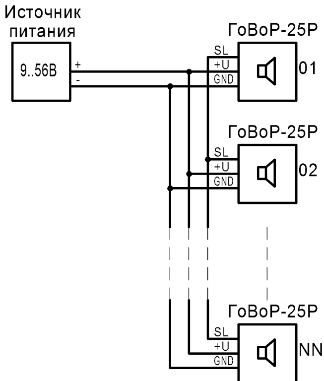
Рис. Б.4 Схема подключения нескольких GoBoP-25P с синхронизацией.
