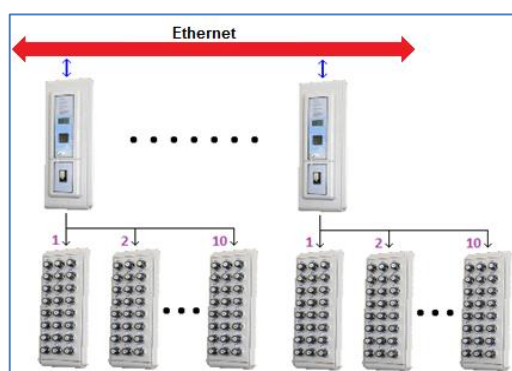
Рисунок 1-17 Схема подключения электронных сейфов для ключей по Ethernet
