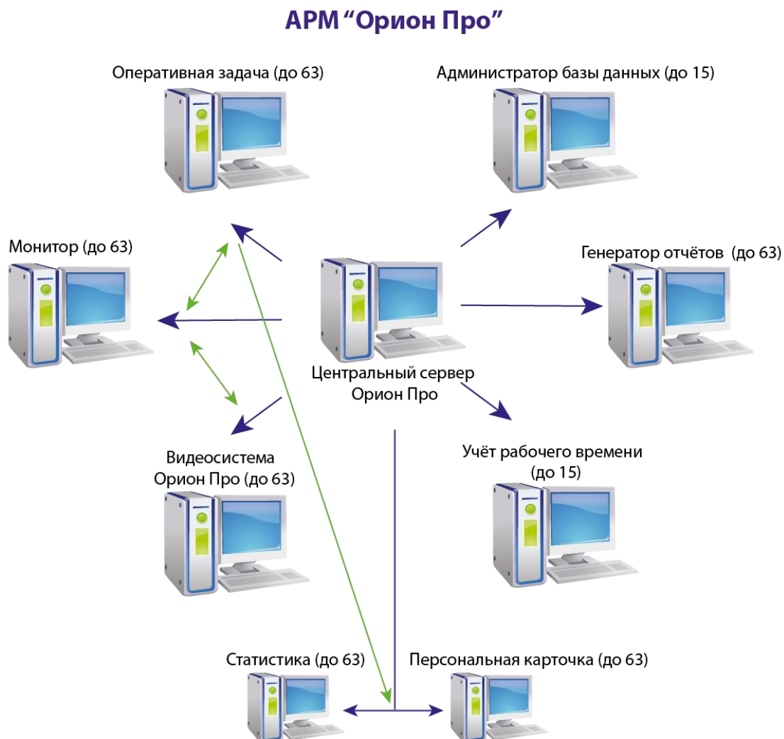
Рисунок 1-1 Схема построения системы на базе АРМ «Орион Про»
