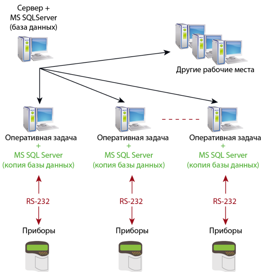
Рисунок 1-20 Система с резервированием
