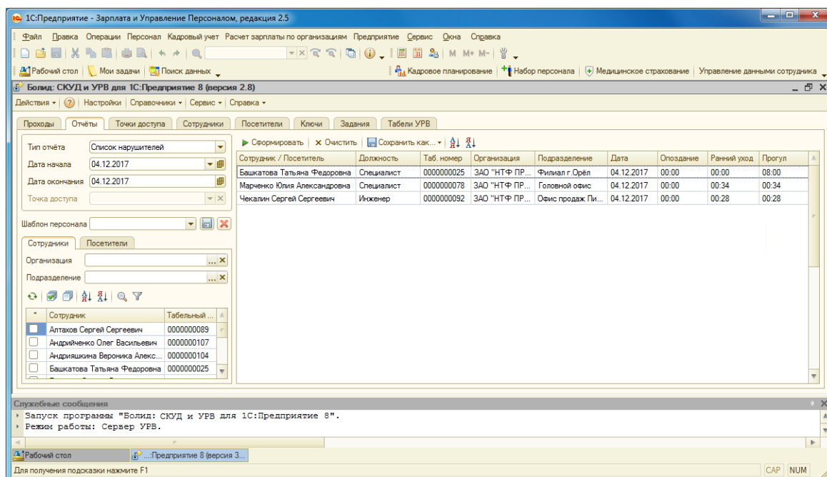
3.13. Список нарушителей.
