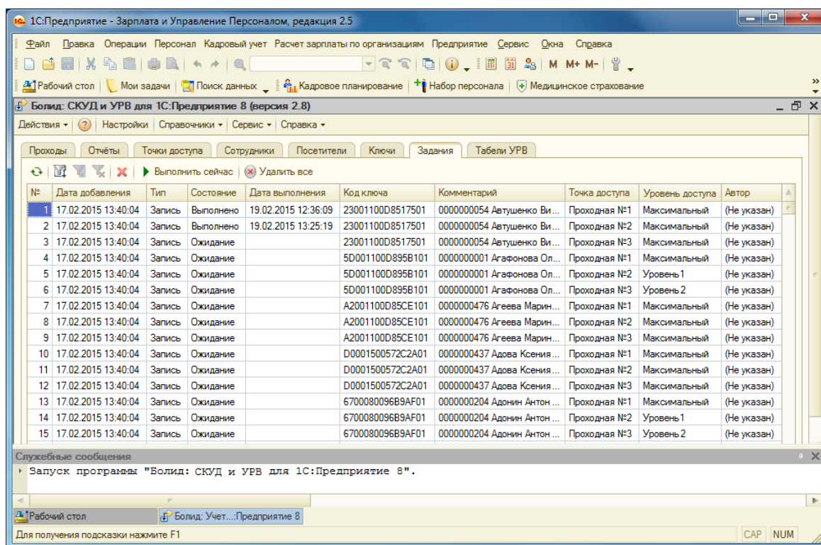
Рисунок 3.26. Страница «Задания».
