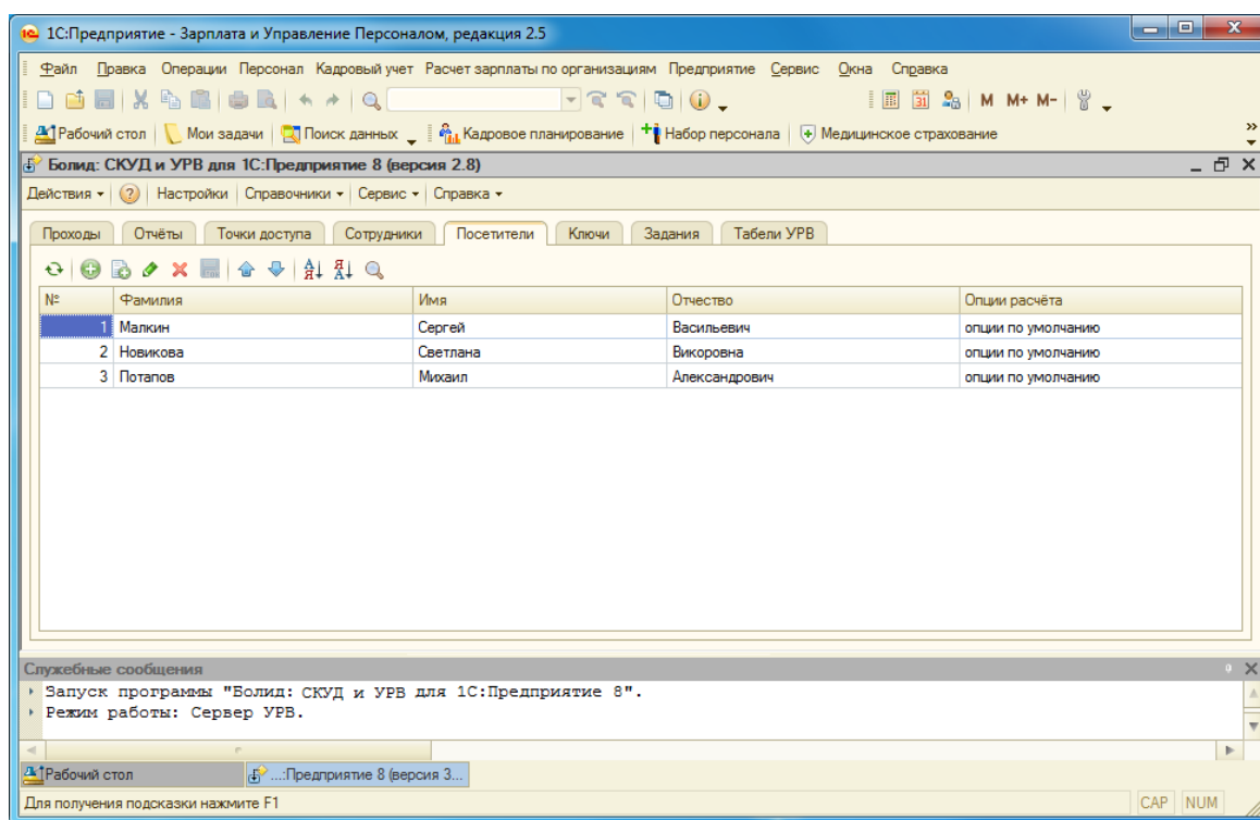
Рисунок 3.22. Страница «Посетители».
