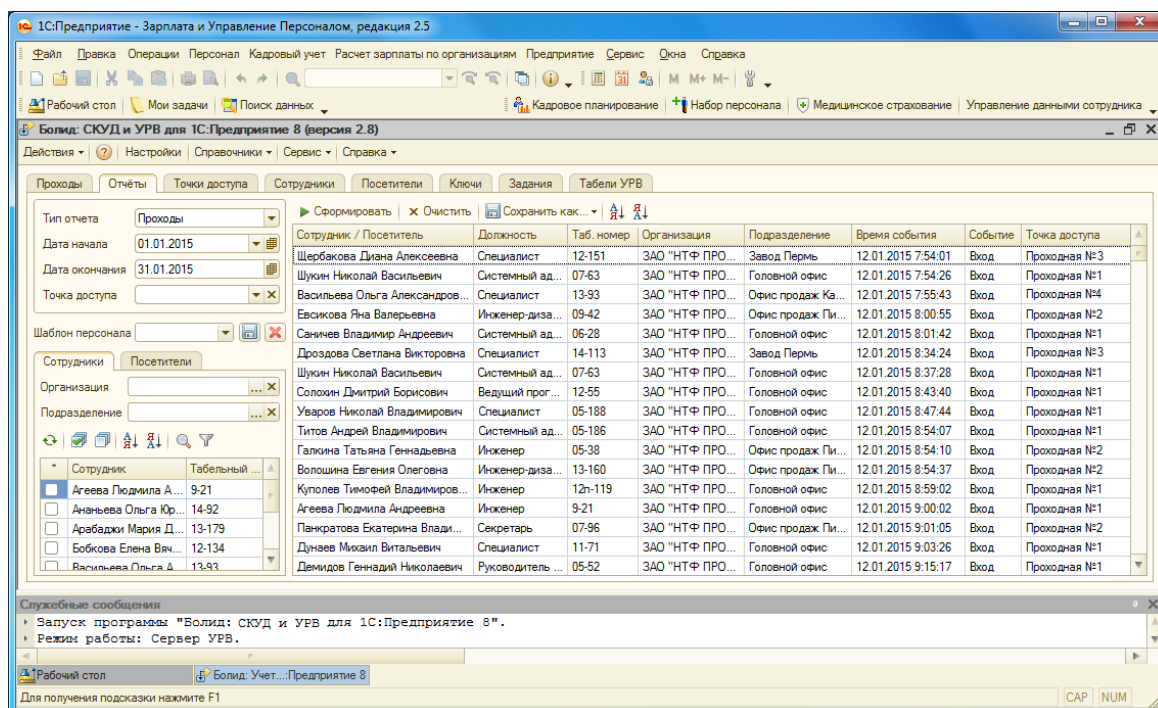
Рисунок 3.10. Проходы.
