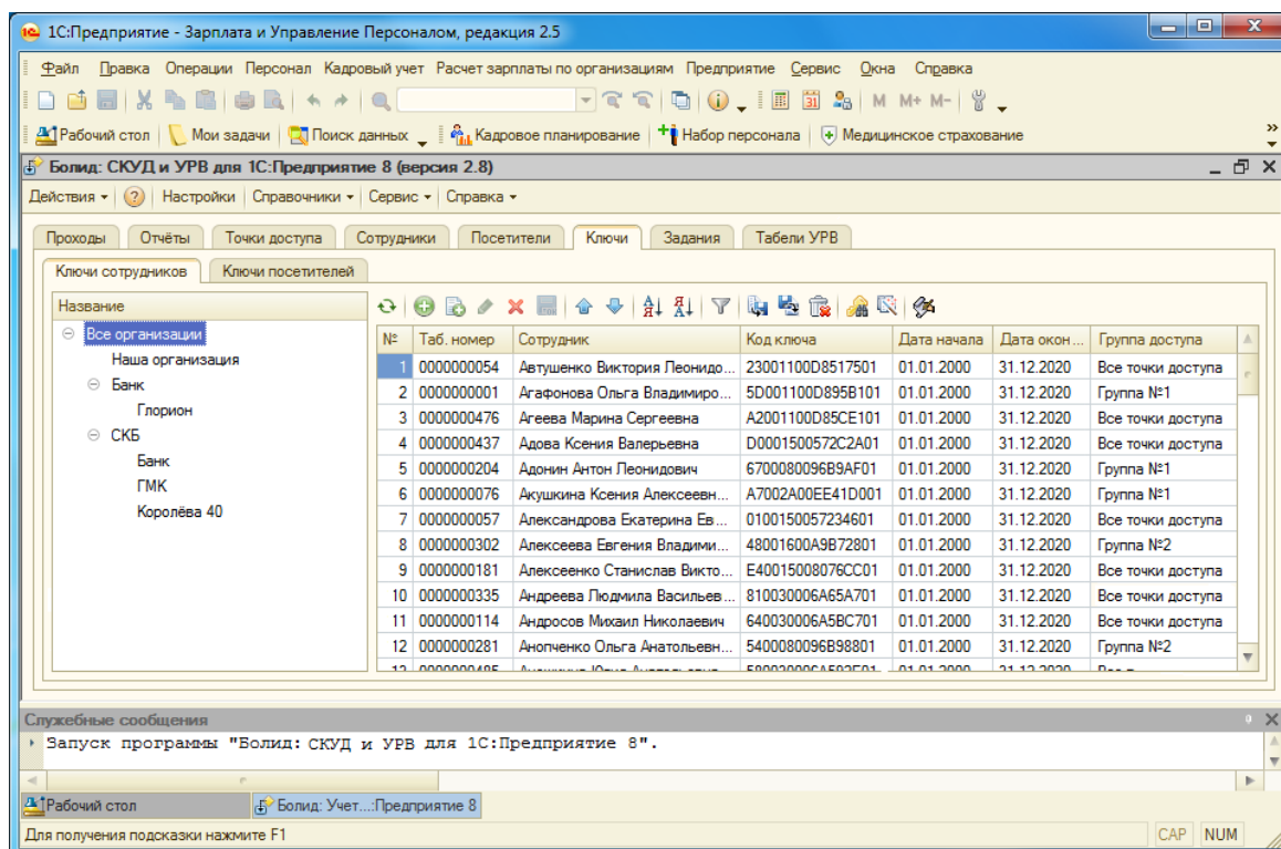
Рисунок 3.24. Страница «Ключи».
