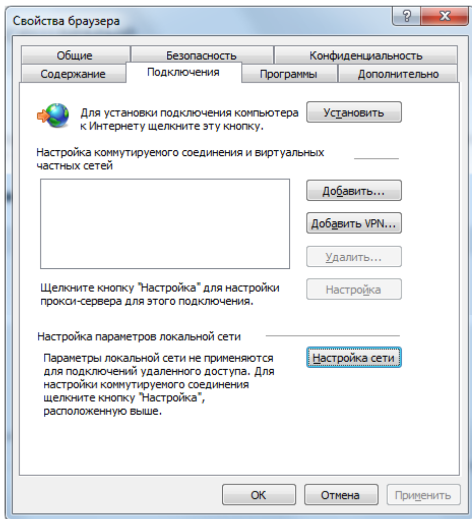
Рисунок 2.10. Настройка сети.
