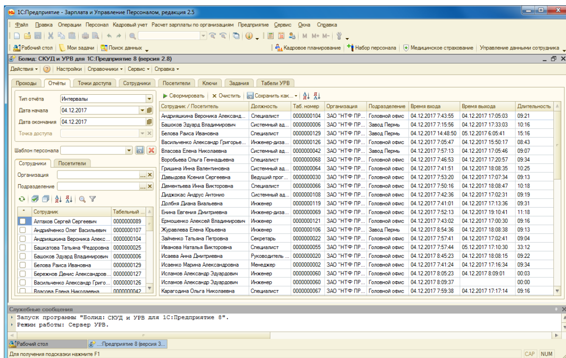
Рисунок 3.11. Интервалы.
