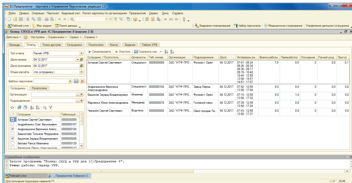
3.14. Расчёт УРВ.
