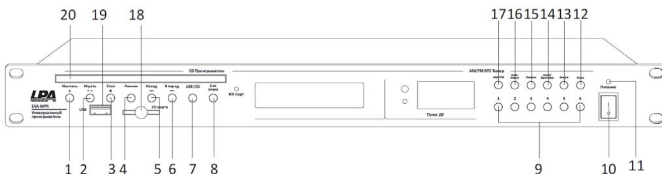
Рис. 3.2. Передняя панель
