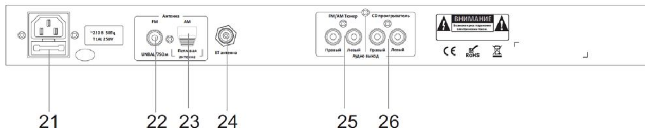
Рис. 3.3. Задняя панель
