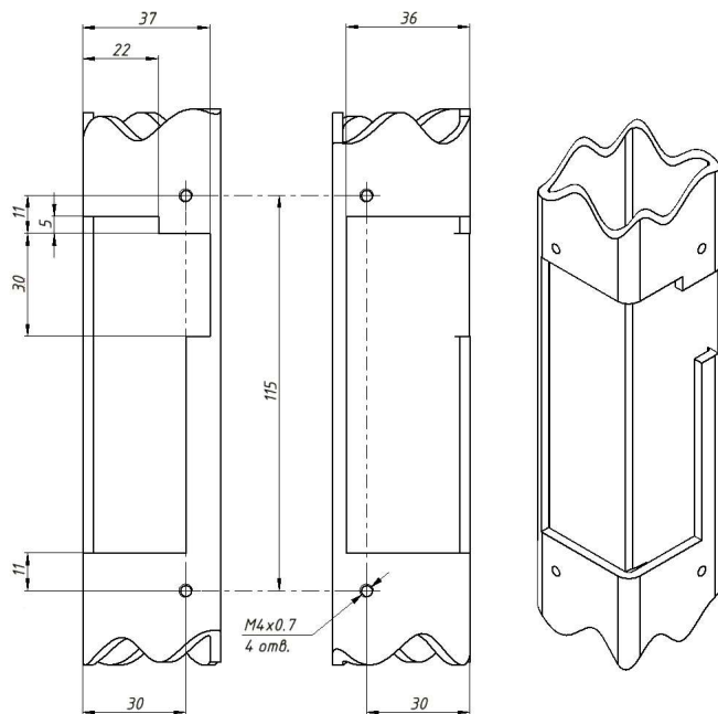
Рис. 2. Размеры необходимых вырезов и расположение отверстий модификаций: Promix-SM330.10.2-01, Promix-SM330.10.3, Promix-SM330.10.3-01
