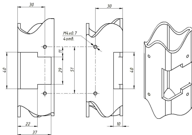
Рис. 1. Размеры необходимых вырезов и расположение отверстий модификации Promix-SM330.10.2
