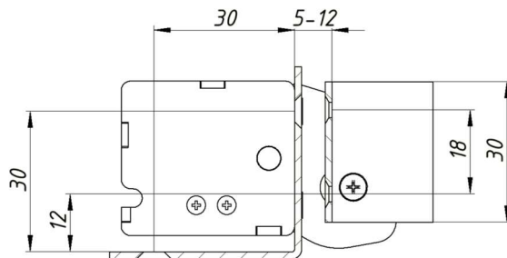
Рис. 3. Взаимное расположение для замка и ригеля модификаций: Promix-SM330.10.2, Promix-SM330.10.2-01, Promix-SM330.10.3, Promix-SM330.10.3-01
