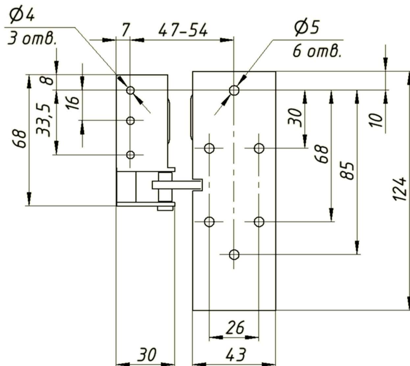
Рис. 4. Габаритные и установочные размеры модификации Promix-SM330.10.3-02
