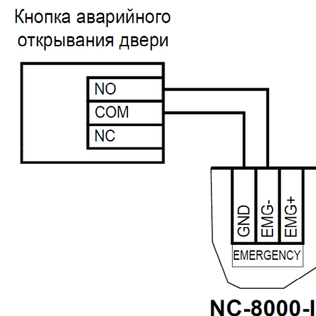
Рисунок 20. Схема подключения кнопки аварийного выхода к одному контроллеру
