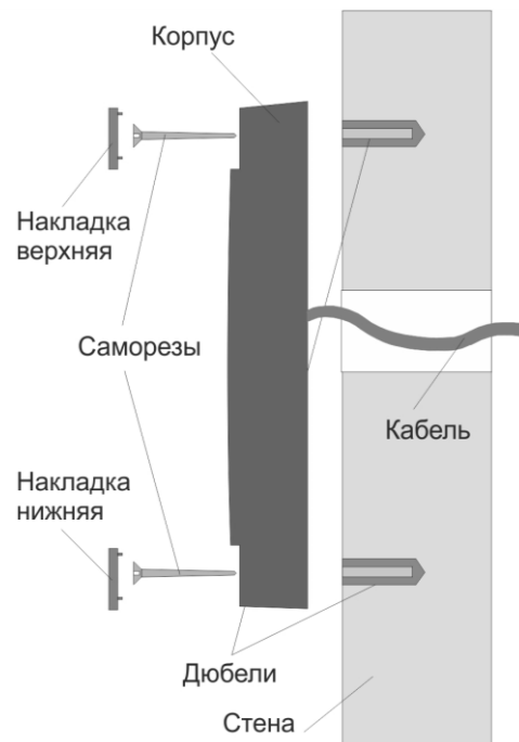
Рисунок 2. Крепление PR-EH16
