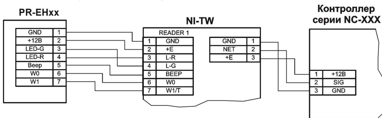
Рисунок 10. Подключение считывателя к контроллеру Parsec через интерфейс NI-TW в режиме Wiegand
