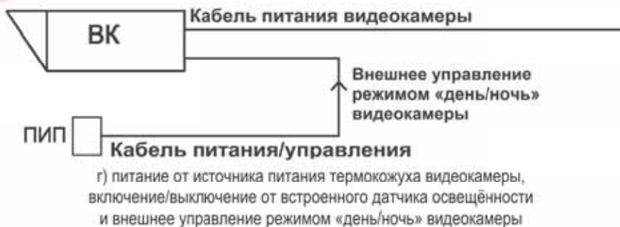
Рисунок 2 – Варианты питания, управления
