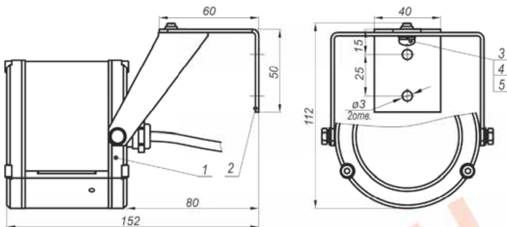
1 – прожектор; 2 – кронштейн; 3 – винт M5x10; 4 – шайба 5; 5 – шайба стопорная 5
