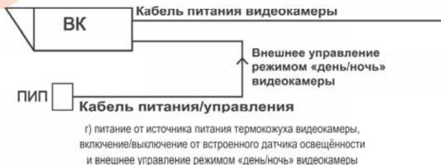
Рисунок 5 – Варианты питания и управления
