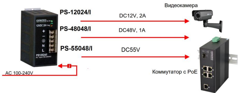
Рис. 4 Подключения блоков питания PS-12024/I, PS-48048/I, PS-55048/I
