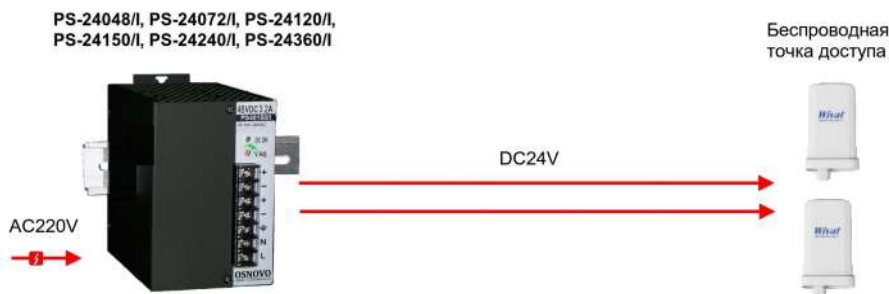
Рис. 7 Подключение PS-24048/I, PS-24072/I, PS-24120/I, PS-24150/I, PS-24240/I, PS-24360/I
