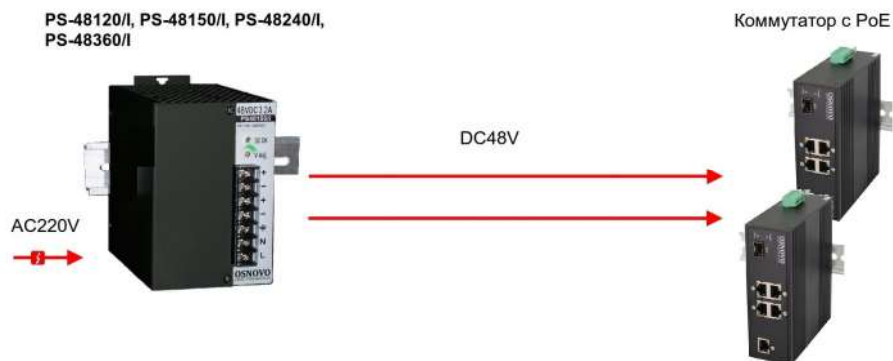
Рис. 8 Подключение PS-48120/I, PS-48150/I, PS-48240/I, PS-48360/I
