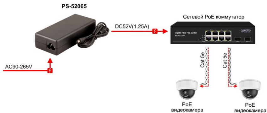
Рис.3 Типовая схема подключения блока питания PS-52065
