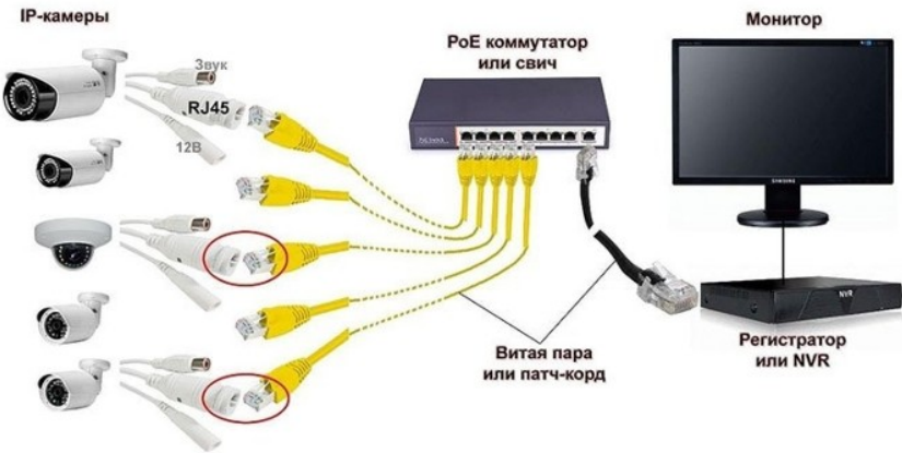
СТАНДАРТНАЯ СХЕМА ПОДКЛЮЧЕНИЯ IP-КАМЕР К РЕГИСТРАТОРУ
