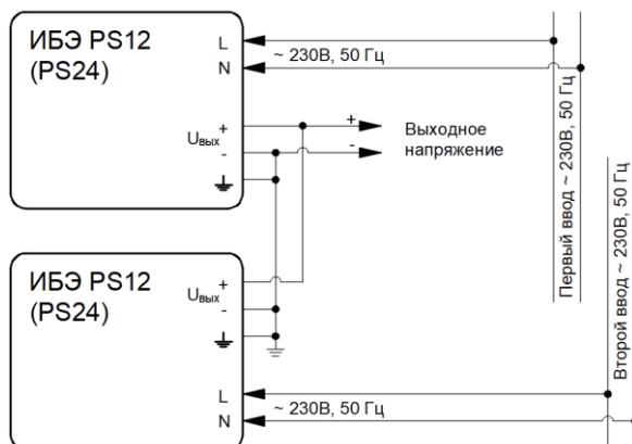
Рис. 6 Бесперебойное питание от двух независимых вводов электропитания 230 В, 50 Гц без применения АКБ.
