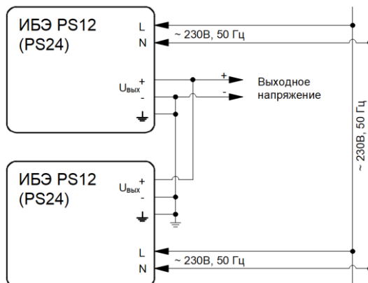
Рис. 5 Параллельное включение ИБЭ для увеличения выходного тока.
