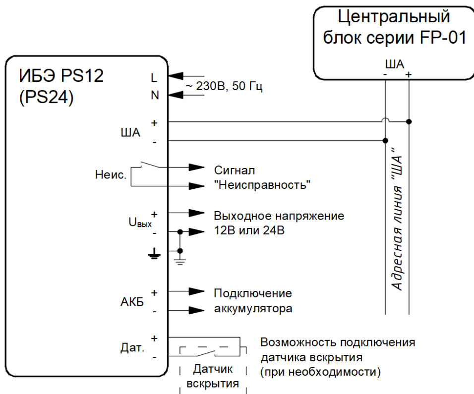
Рис. 1. Схема подключения ИБЭ.
