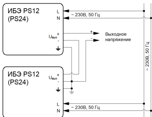
Рис. 4 Последовательное включение ИБЭ для увеличения выходного напряжения.
