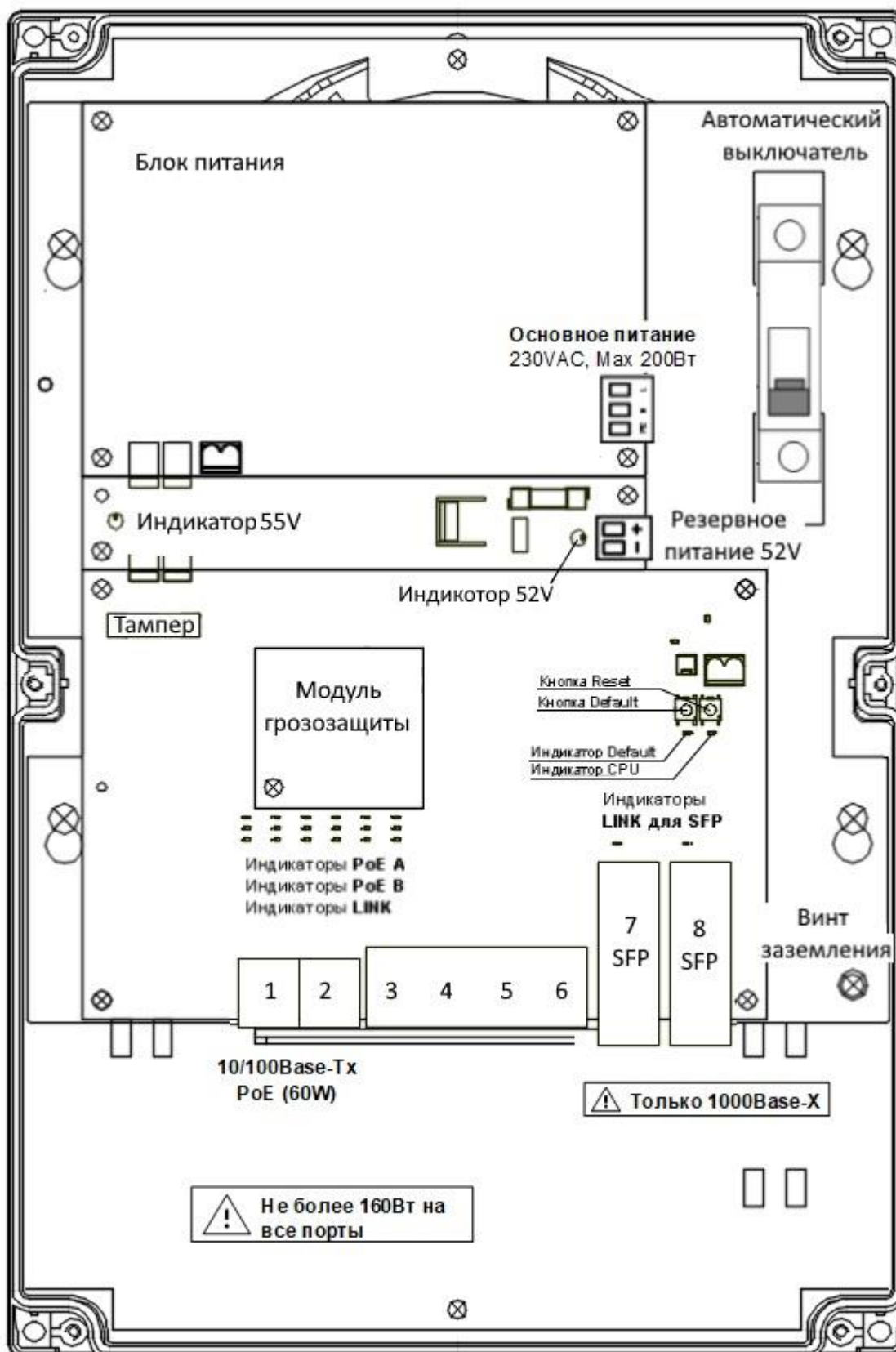
Рисунок 3.2 - Расположение элементов коммутатора PSW -2G6F+
