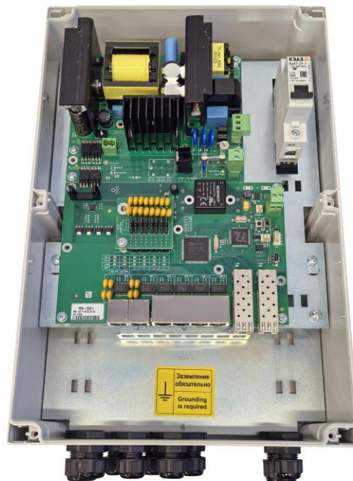
Рисунок 3.1.2 – Вид без крышки
