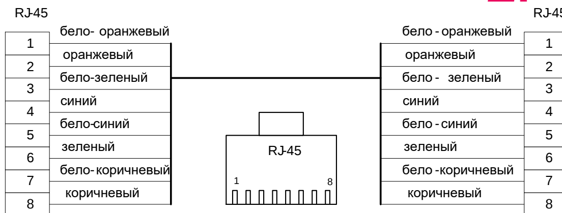
Рисунок 7.6 - Разделка кабеля.
