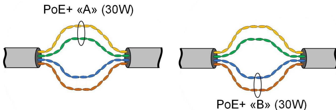
Рисунок 3.3 - Схема питания по PoE для разных случаев
