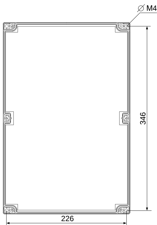
Рисунок 7.1 - Разметка крепления
