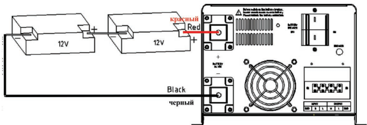
Схема подключения аккумуляторных батарей U=24В. Модель PSW-HW 2500–3500 Вт
