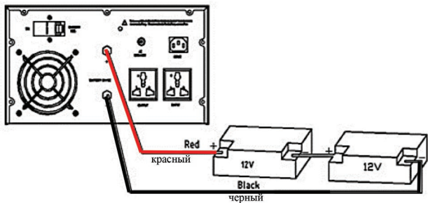
Схема подключения аккумуляторных батарей U=24В. Модель PSW-H 1600 Вт
