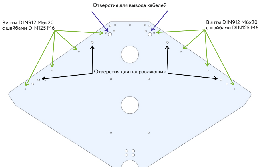
Рисунок 9.7 - Крыша зоны прохода
