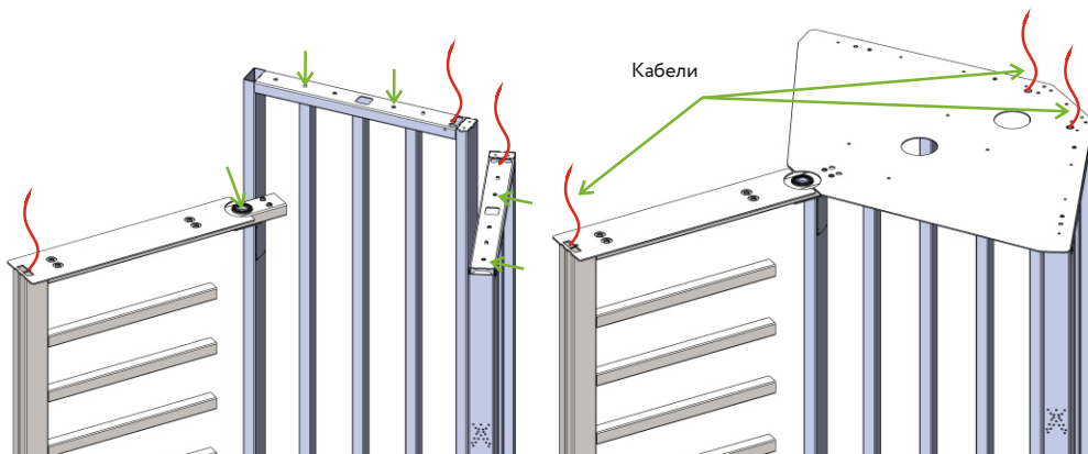
Рисунок 9.8 - Турникет с установленной крышей зоны прохода
