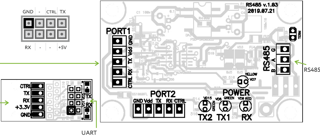
Рисунок 5.2 - Плата RS485
