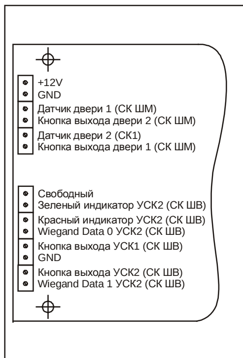
Рис. 2 Колодка подключения ПУ
