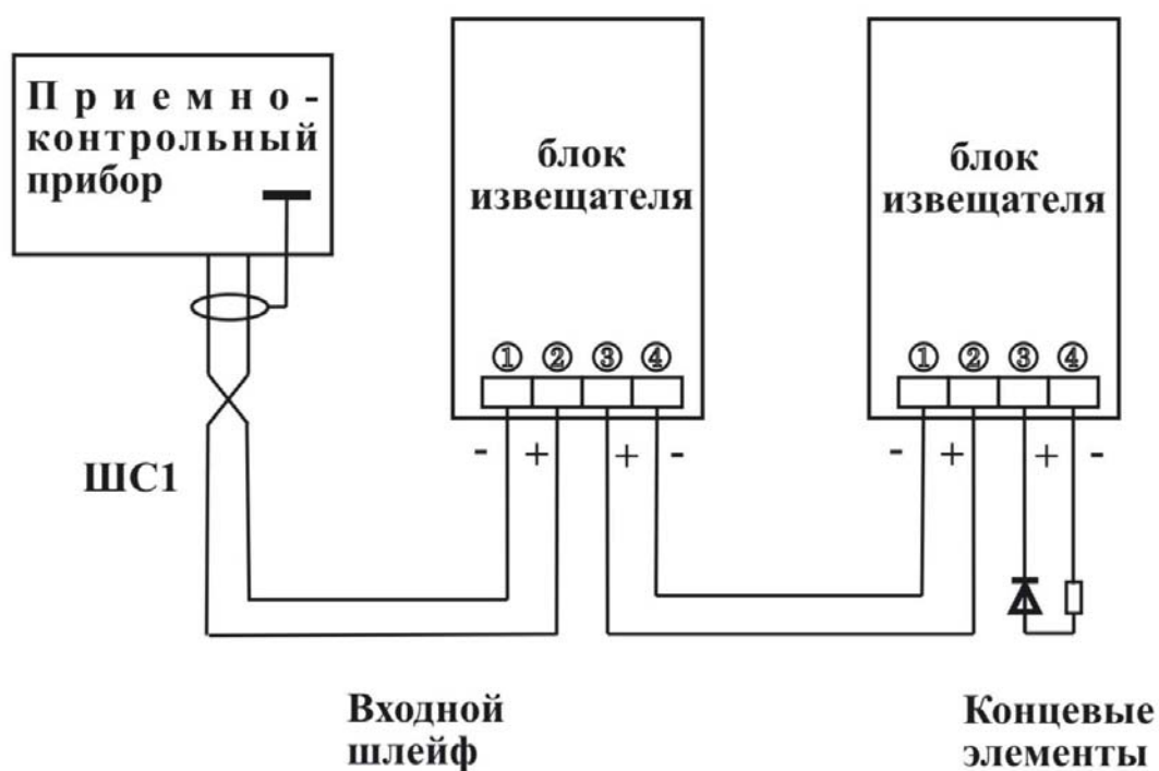
Рис 8 Схема подключения нескольких извещателей Пульсар 1-01 в один шлейф приемно- контрольного прибора
