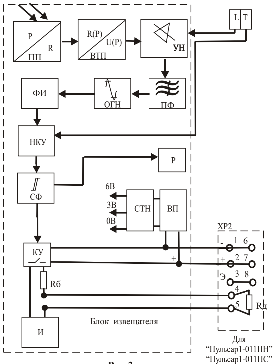
Рис 3 Схема функциональная
