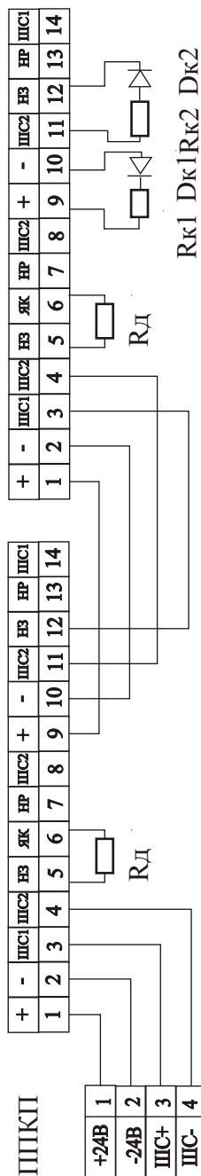
Рис. 7а Монтажная схема последовательного подключения “Пульсар1-011ПНК”, “Пульсар1-011ПСК” с нормально замкнутым контактом реле
