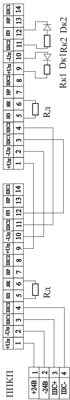
Рис. 7а Монтажная схема последовательного подключения “Пульсар3-014НК”, “Пульсар3-014СК” с нормально замкнутым контактом реле.
