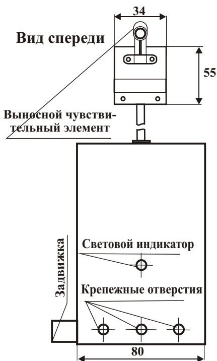
Рис 4 Извещатель пожарный пламени “Пульсар 4-011Н” со снятой розеткой
