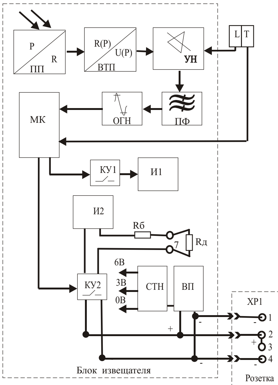
Рис 7 Схема функциональная
