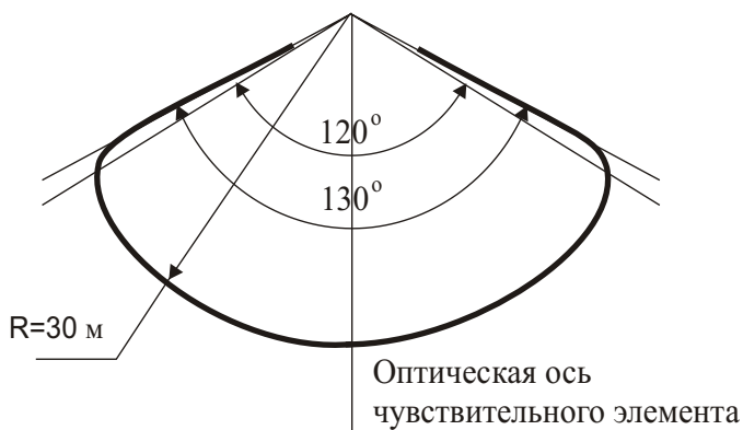
Рис 5 Проекция поля зрения чувствительного элемента извещателя
