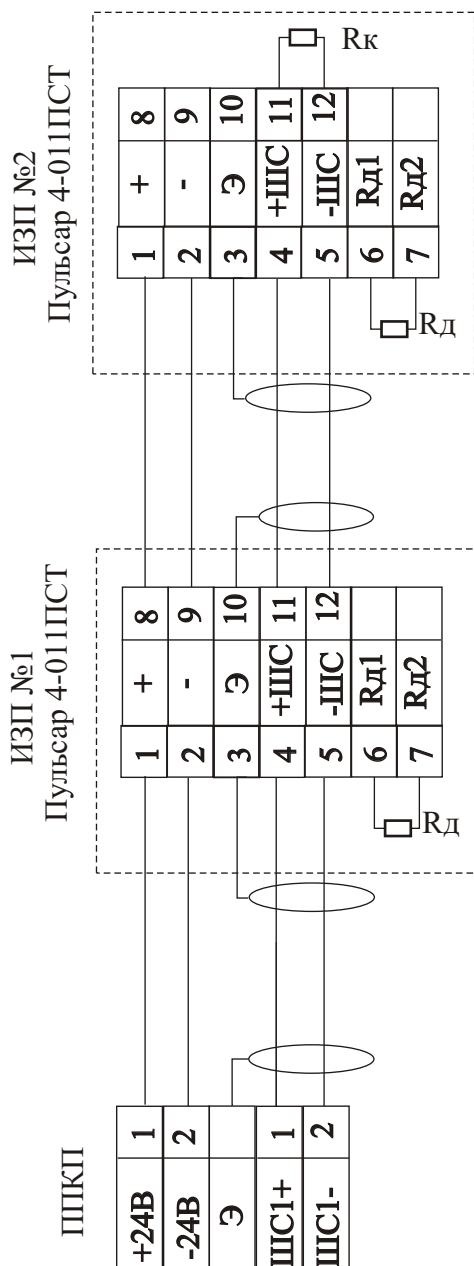
Рис. 56 Схема подключения извещателей “Пульсар4-011ПНТ” “Пульсар4-011ПСТ” к ППКП
