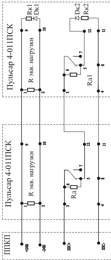
Рис. 7б Принципиальная схема последовательного подключения “Пульсар4-011ПНК”, “Пульсар4-011ПСК” с нормально замкнутым контактом реле
