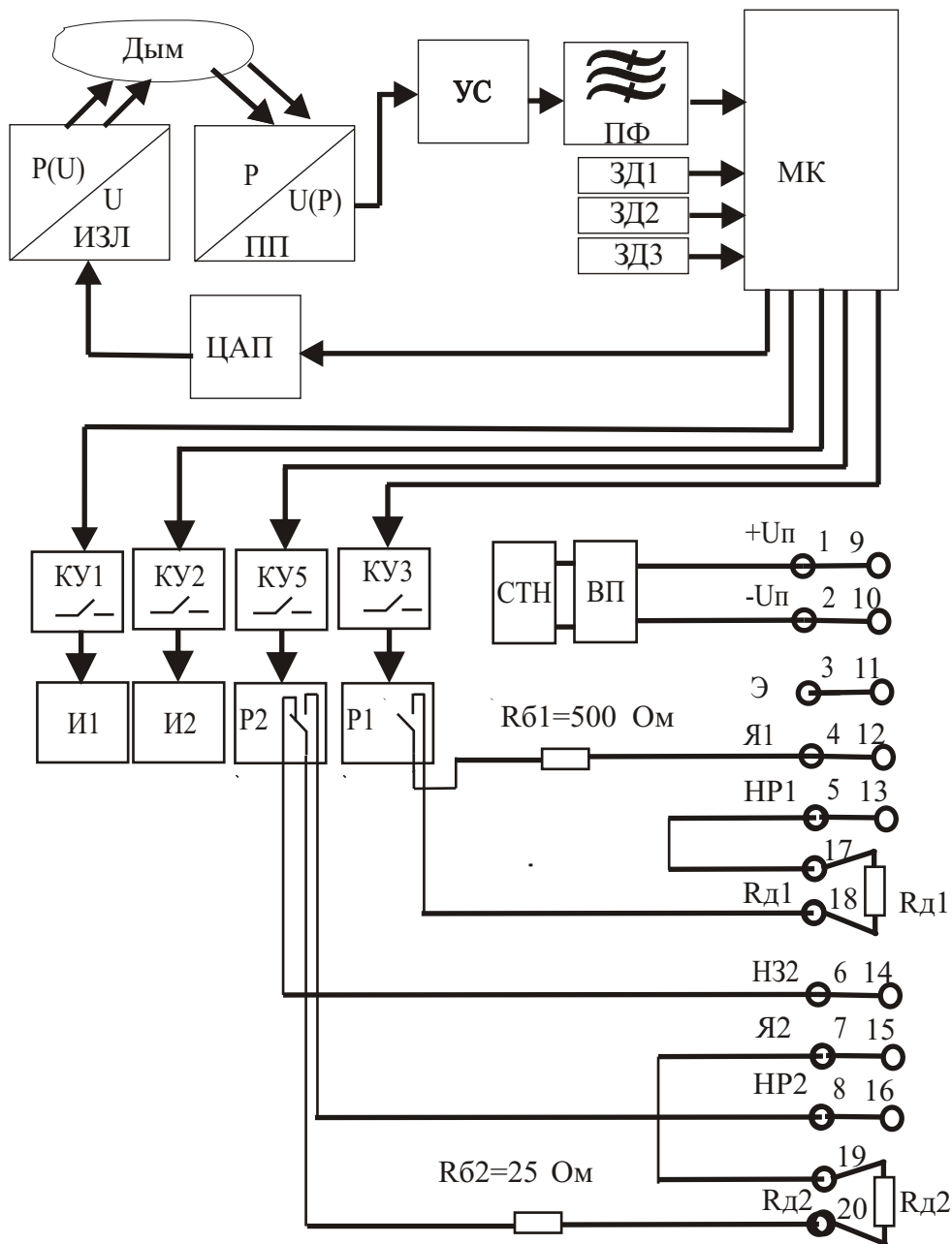
Рис. 2. Схема функциональная извещателя “Пульсар 52K2(В,Д)”.
