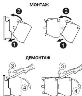
Монтаж и демонтаж контактных блоков
