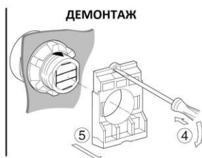
Монтаж и демонтаж кнопки
