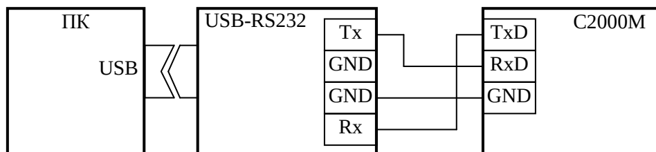
Рисунок 6 Простейшая схема подключения пульта «C2000M» при конфигурировании персональным компьютером по интерфейсу RS-232, а также при использовании его в качестве преобразователя интерфейсов RS-232 – RS-485
