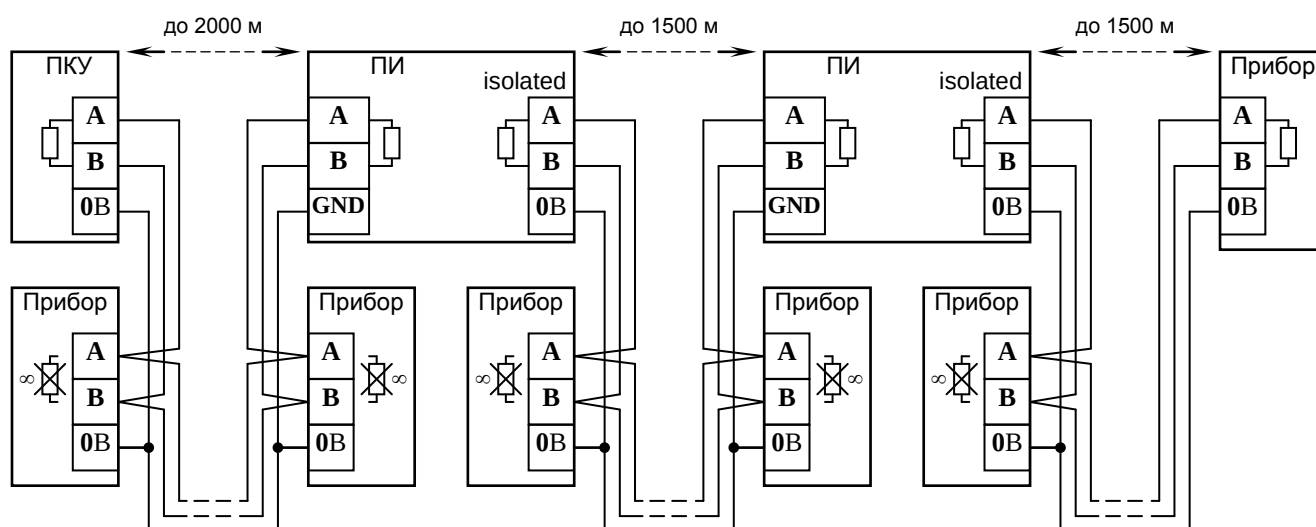
Рисунок 3 Схема подключения приборов к магистральному интерфейсу RS-485
