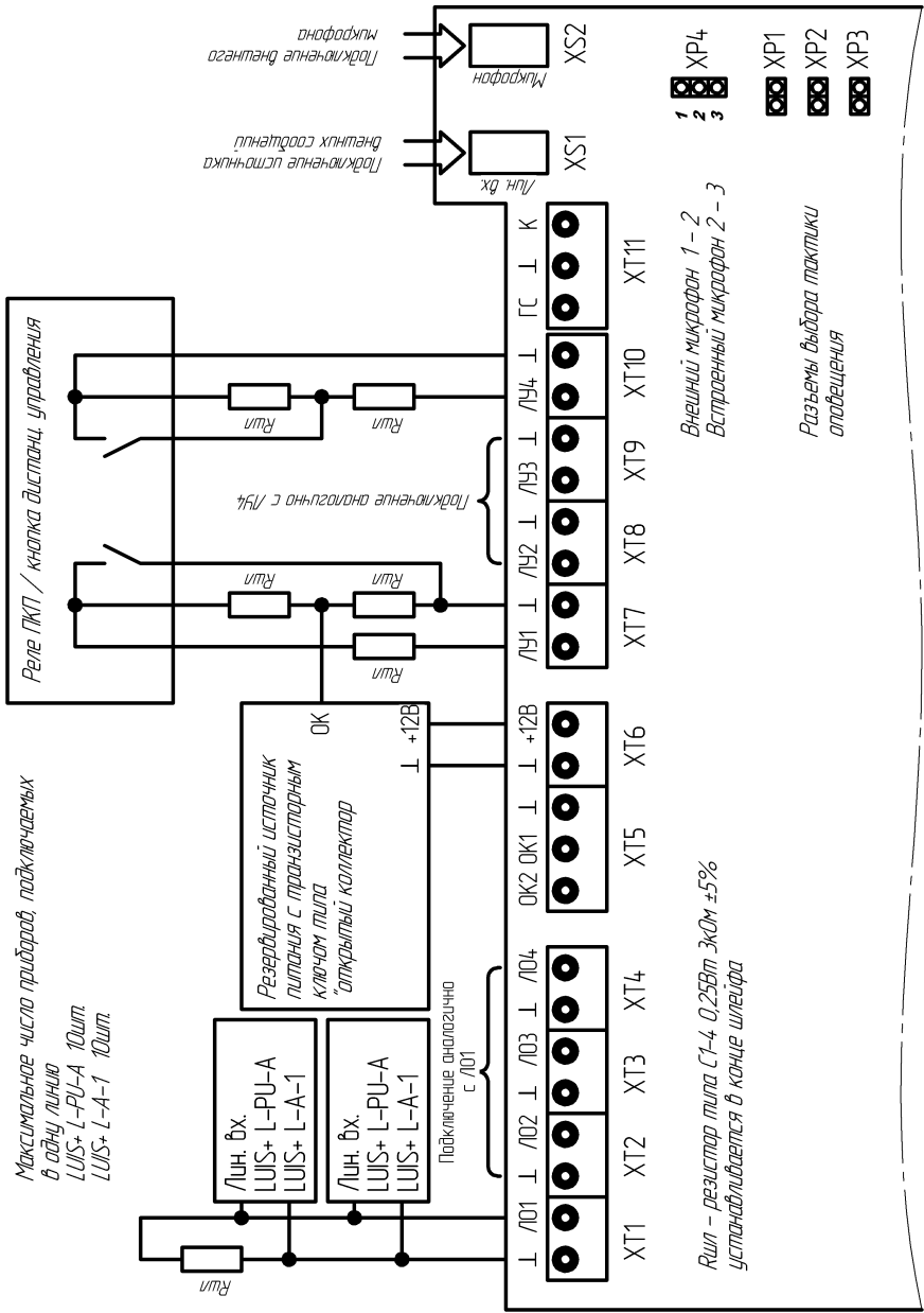
Рисунок-1 Схема внешних подключений прибора LUIS+ L-PU-LT с вариантом реализации запрета трансляции с линейного входа (см. п.п. 4.2) при питании прибора LUIS+ L-PU-LT от резервированного источника питания с транзисторным ключом типа «открытый коллектор»
