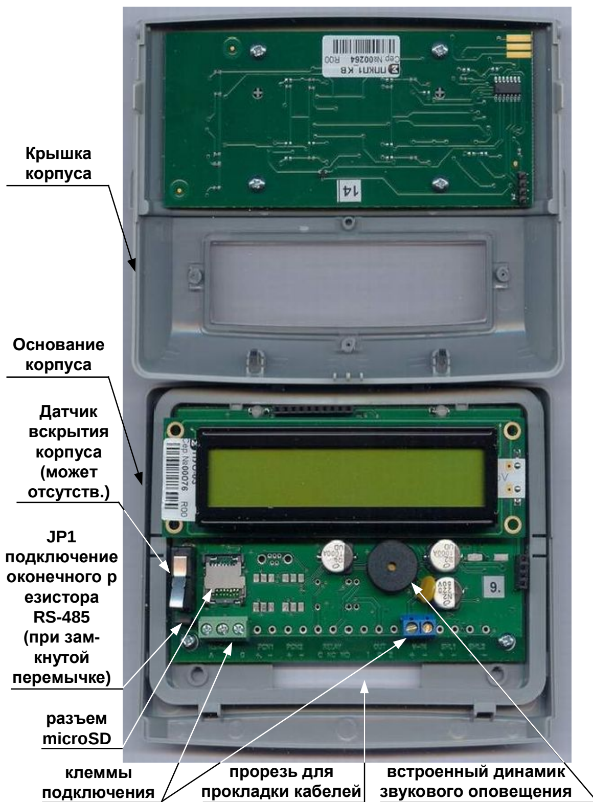
Рис. 3 Основание и крышка корпуса
