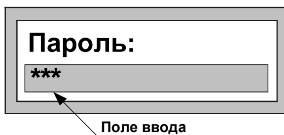
Рис. 9 Авторизация пользователя
