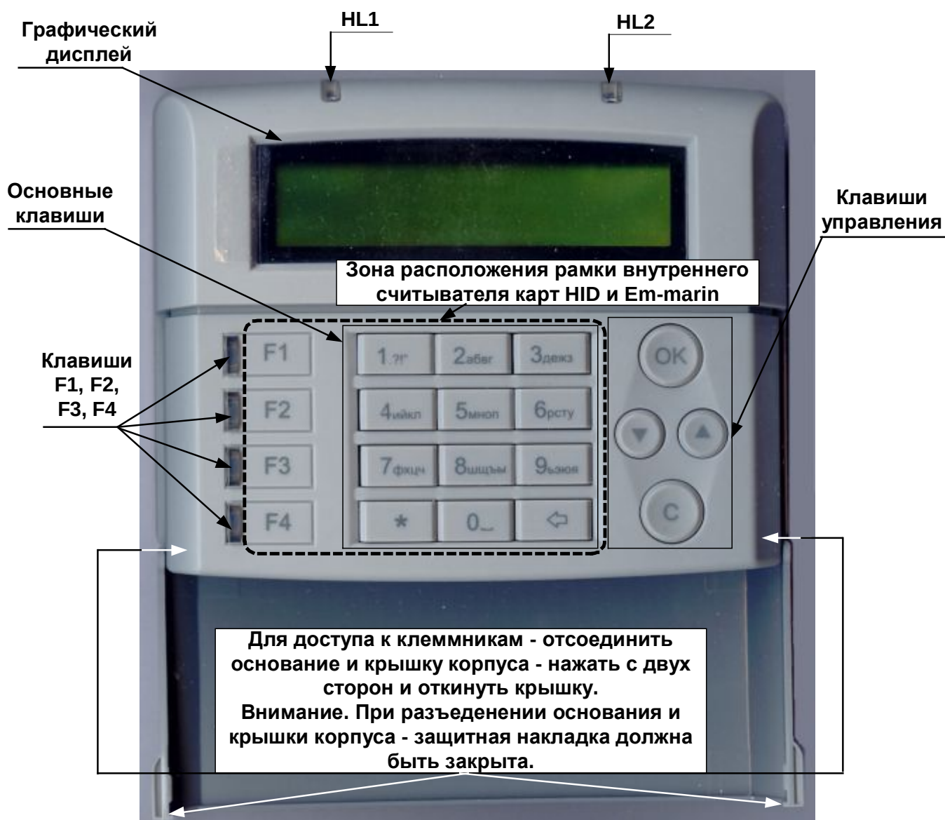
Рис. 1 Внешний вид ПУО
