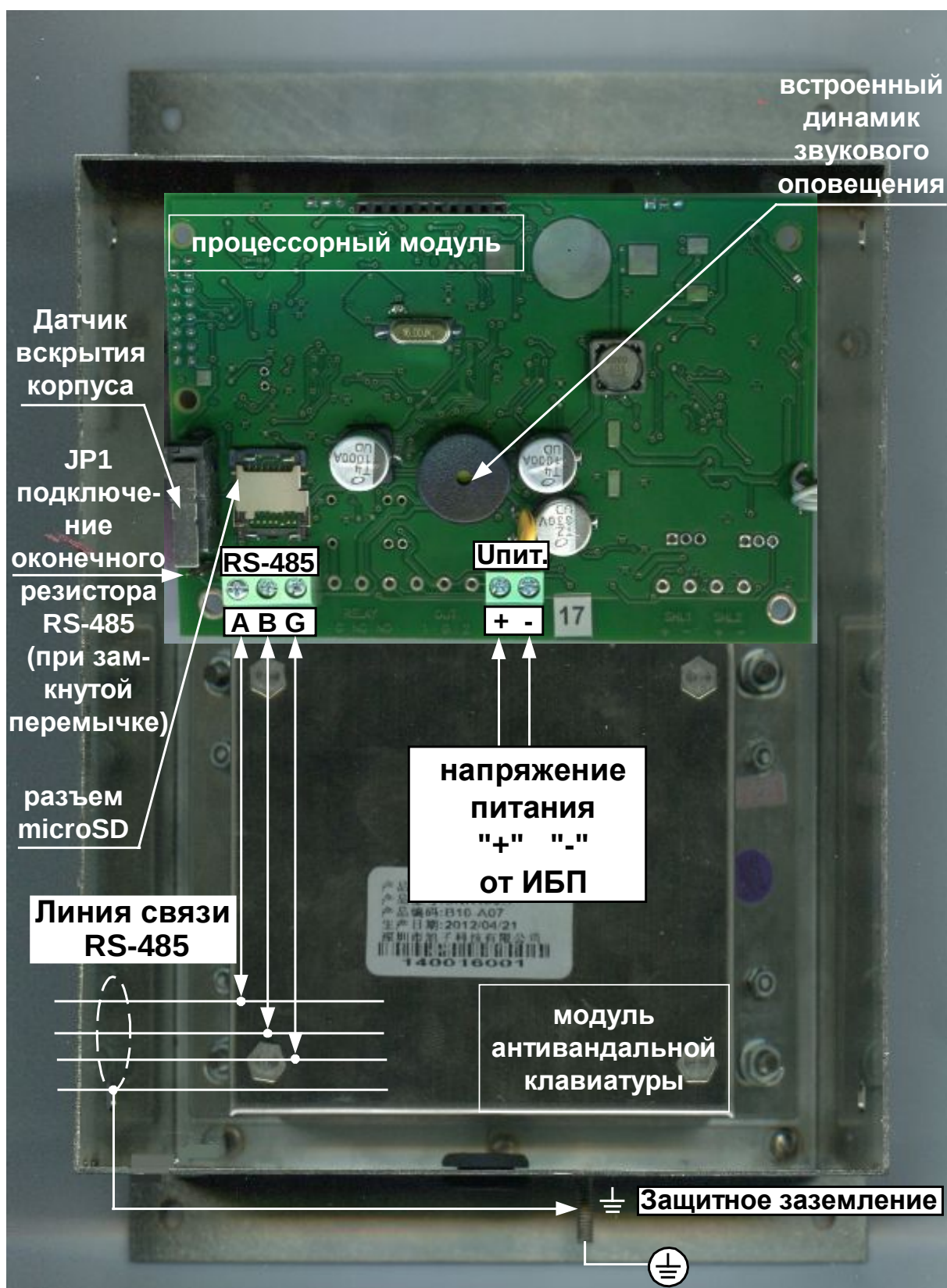
Рис. 2 Расположение элементов, подключение (вид без дна корпуса)
