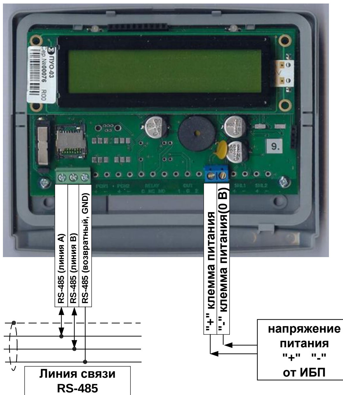
Рис. 7 Подключение ПУО
