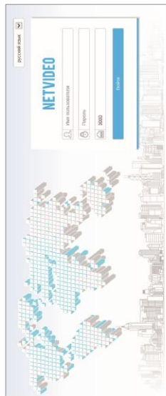
Рис. 1 Интерфейс входа
