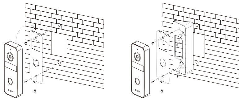
Порядок монтажа
