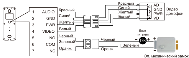
Подключение электромеханического замка
