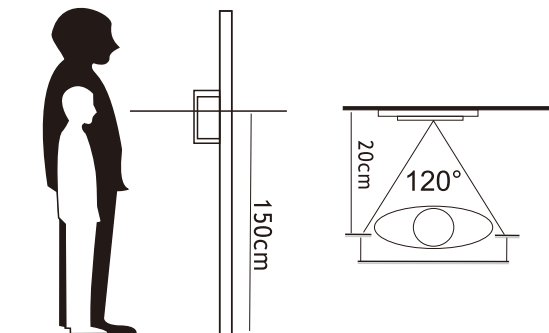
Схема монтажа
