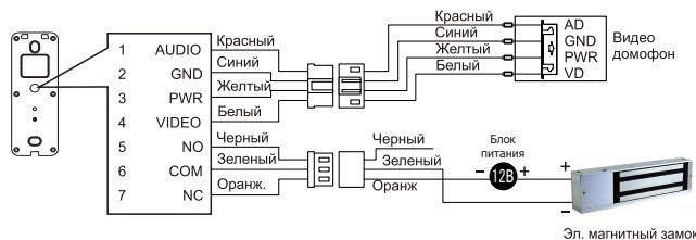
Подключение электромагнитного замка
