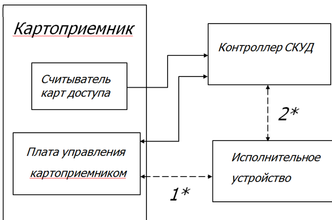
Рисунок 17 – Структурная схема №3
