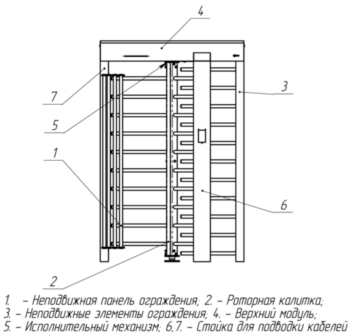
Рисунок 5 – Общий вид турникета
