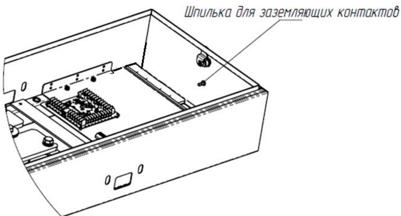
Рисунок 17 – Расположение шпилек в верхнем модуле
