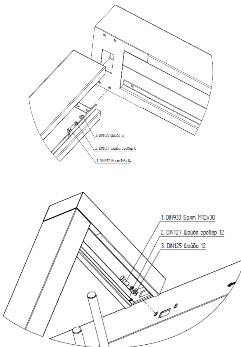
Рисунок 7 – Установка неподвижного элемента ограждения
