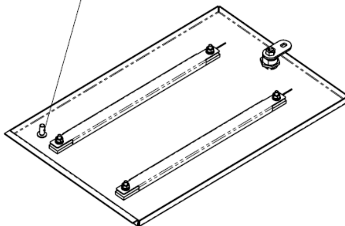
Рисунок 20 – Расположение шпилек в лючке
