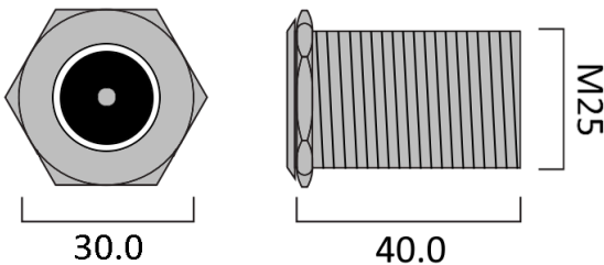
Рис.1 Габариты QR-X-2.
