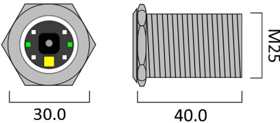
Рис.2 Габариты QR-X-6.
