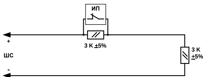
Рис. 6 Пожарный ШС с пассивным ИП (при срабатывании одного ИП формируется извещение «Пожар»)
