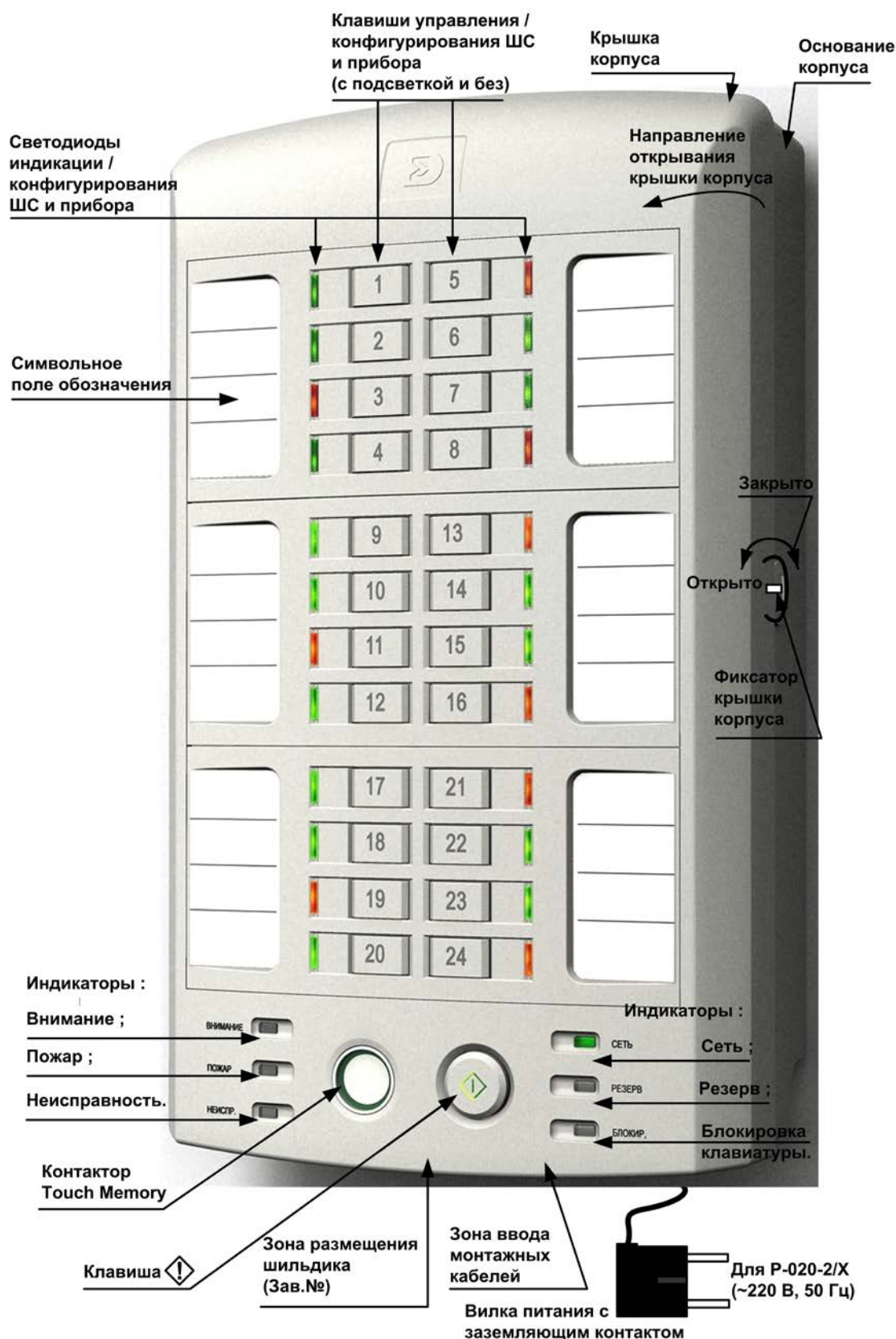
Рис. 1 Внешний вид приборов Р-020-1 и Р-020-2 (внешний вид прибора “ Р-020-М ” – см. Приложение Е, вместо кнопки ⚠ введена кнопка “Подтверждение”)
